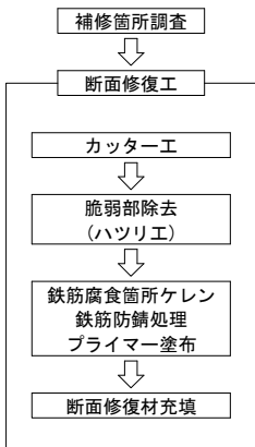
施工手順
