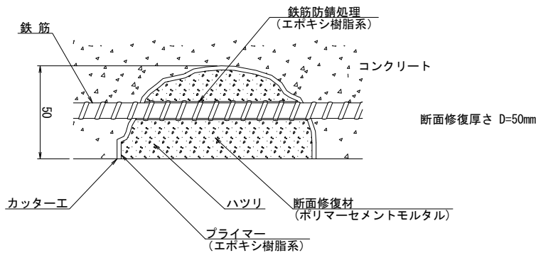
左官工法
