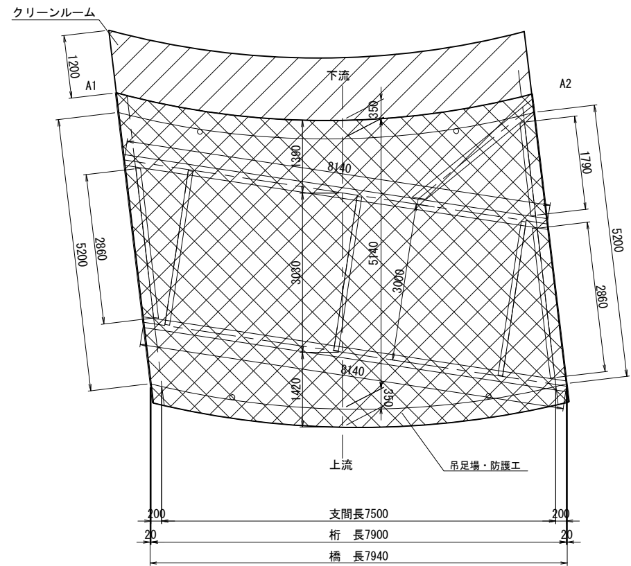
平面図 S=1:50
