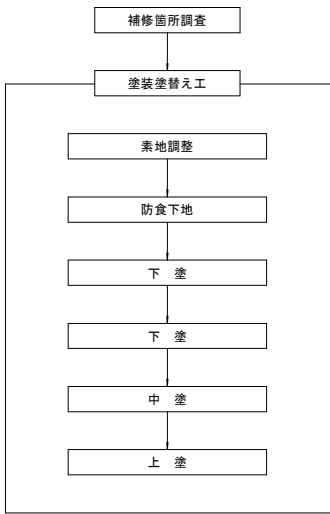
施工手順
