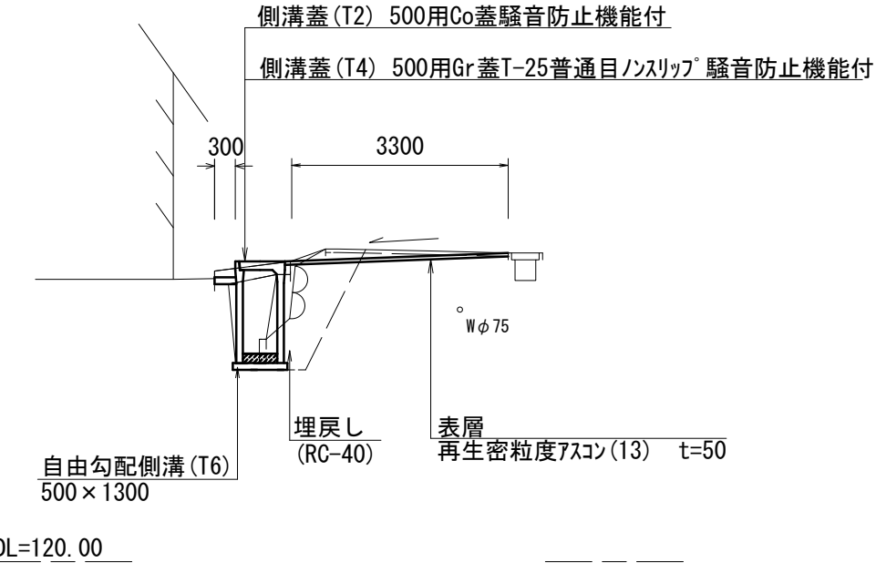
No. 0+14. 9 (同所) ～No. 0+16. 9
