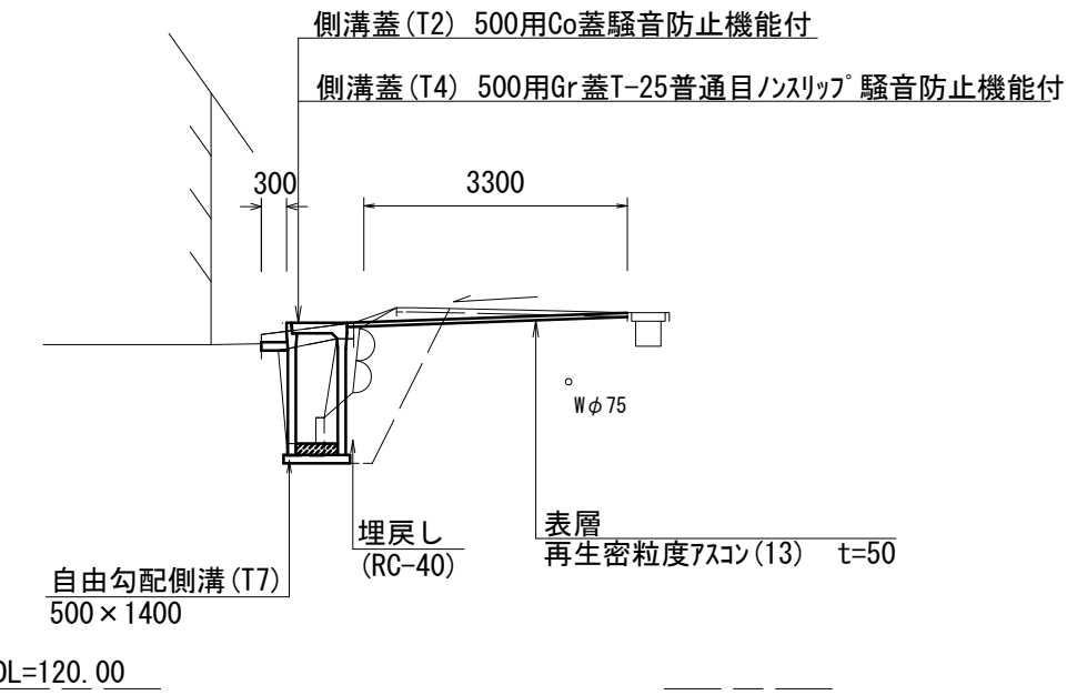
No. 0+16. 9 (同所) ～No. 0+17. 9
