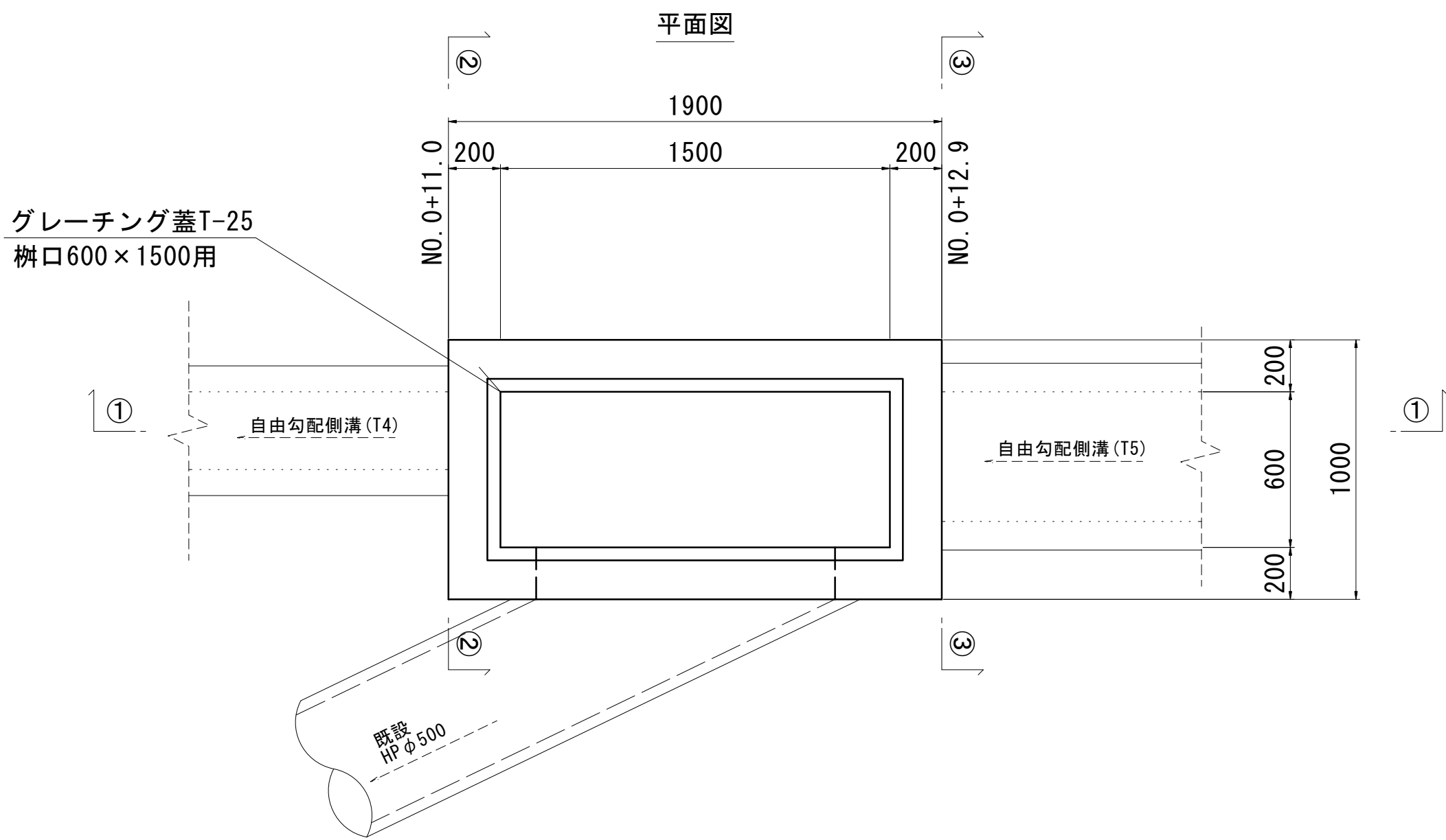
現場打集水桝(T1) (600×1500×1250) S=1:20
