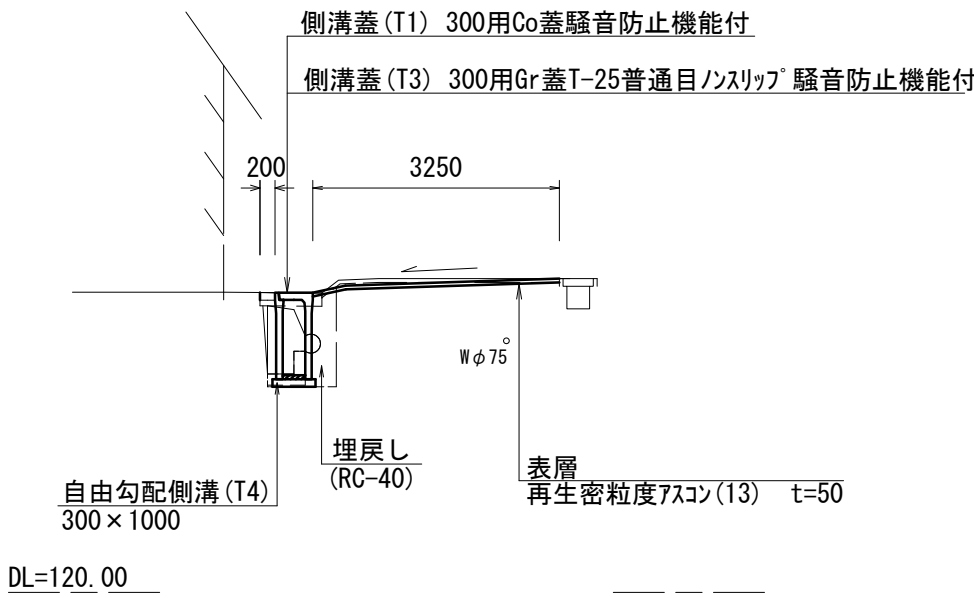
No. 0+7. 0 (同所) ～No. 0+12. 9
