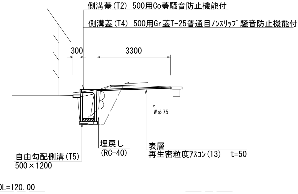
No. 0+12. 9 (同所) ～No. 0+14. 9
