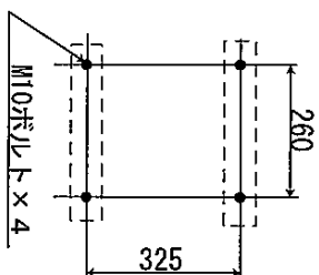
アンカー寸法図
