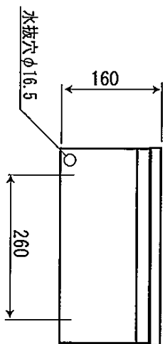
底面図
