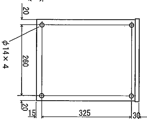
背面図
