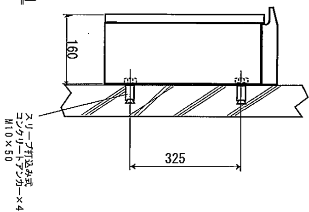
アンカー寸法図
