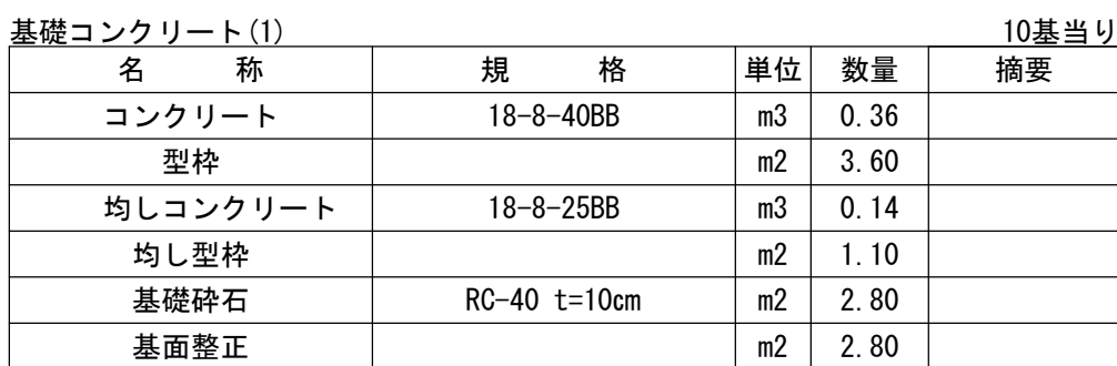
作業土工 10基当り 名 称 規 格 単位 数量 摘要 床掘り 土砂 m3 4.83 埋戻し 流用土 m3 4.05
