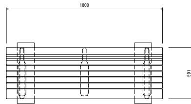
平面図 S=1:15
