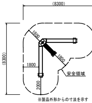
安全領域図
