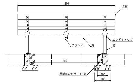
立面図 S=1:15
