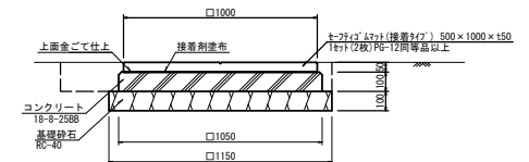
B-B 断面图
