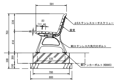
側面図 S=1:15
