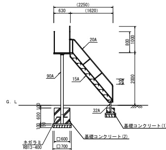
A 矢視区
