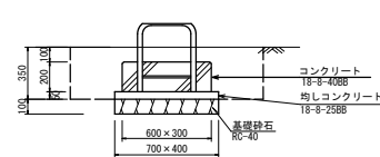
基礎コンクリート(1)
