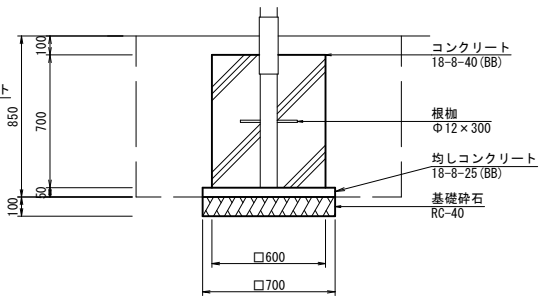
コンクリート基礎 (4) S=1:20
