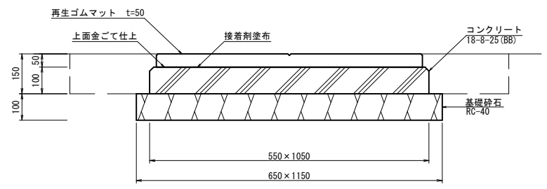
断面図 S=1:10
