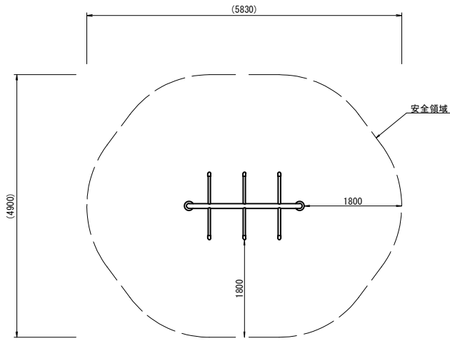
安全領域図 S=1:50
