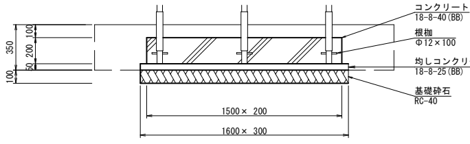
コンクリート基礎 (3) S=1:20
