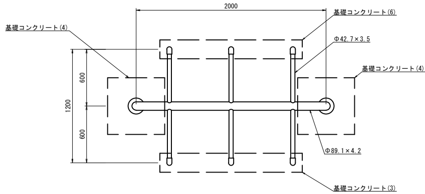
平面図 S=1:20
