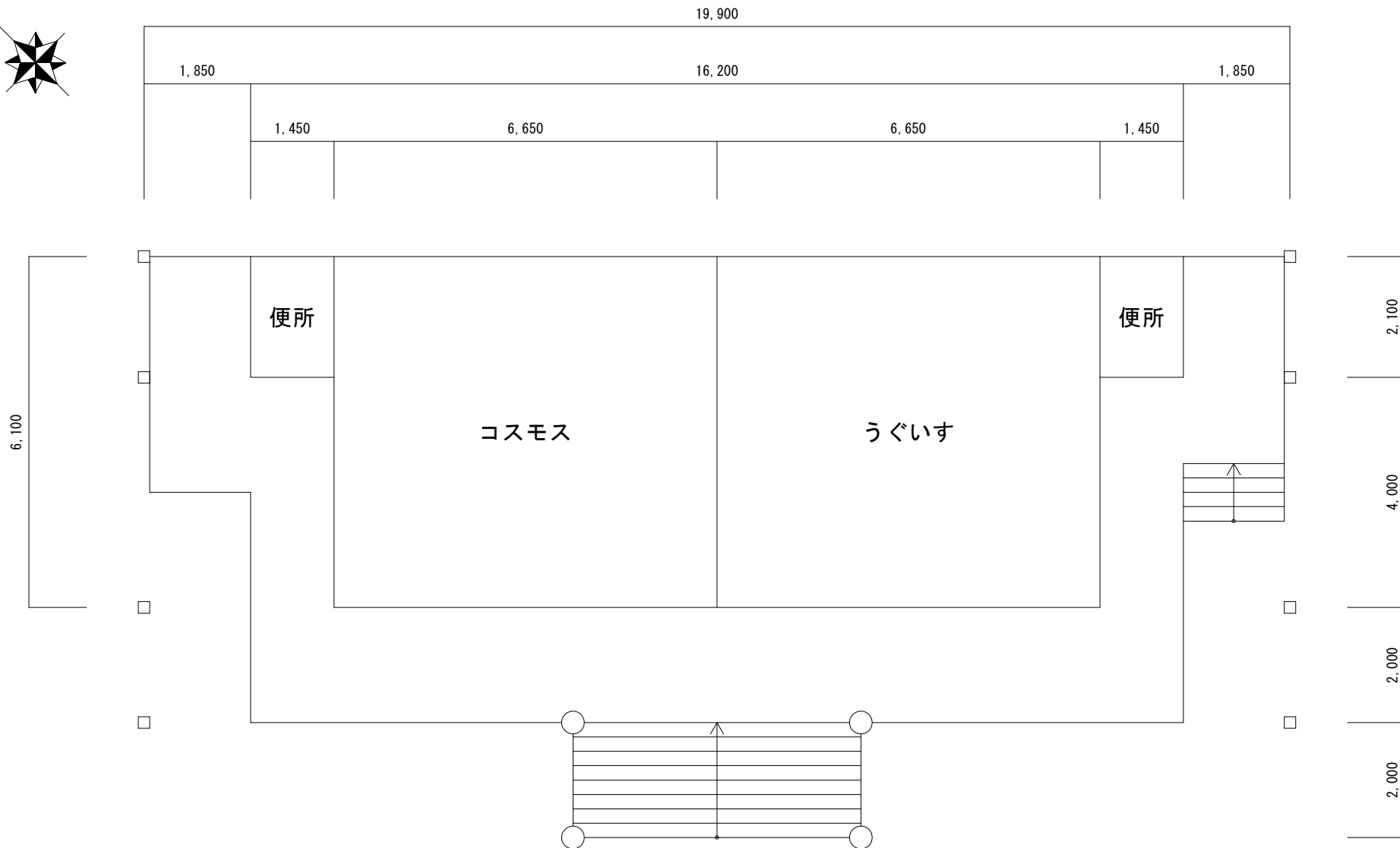
平面図
