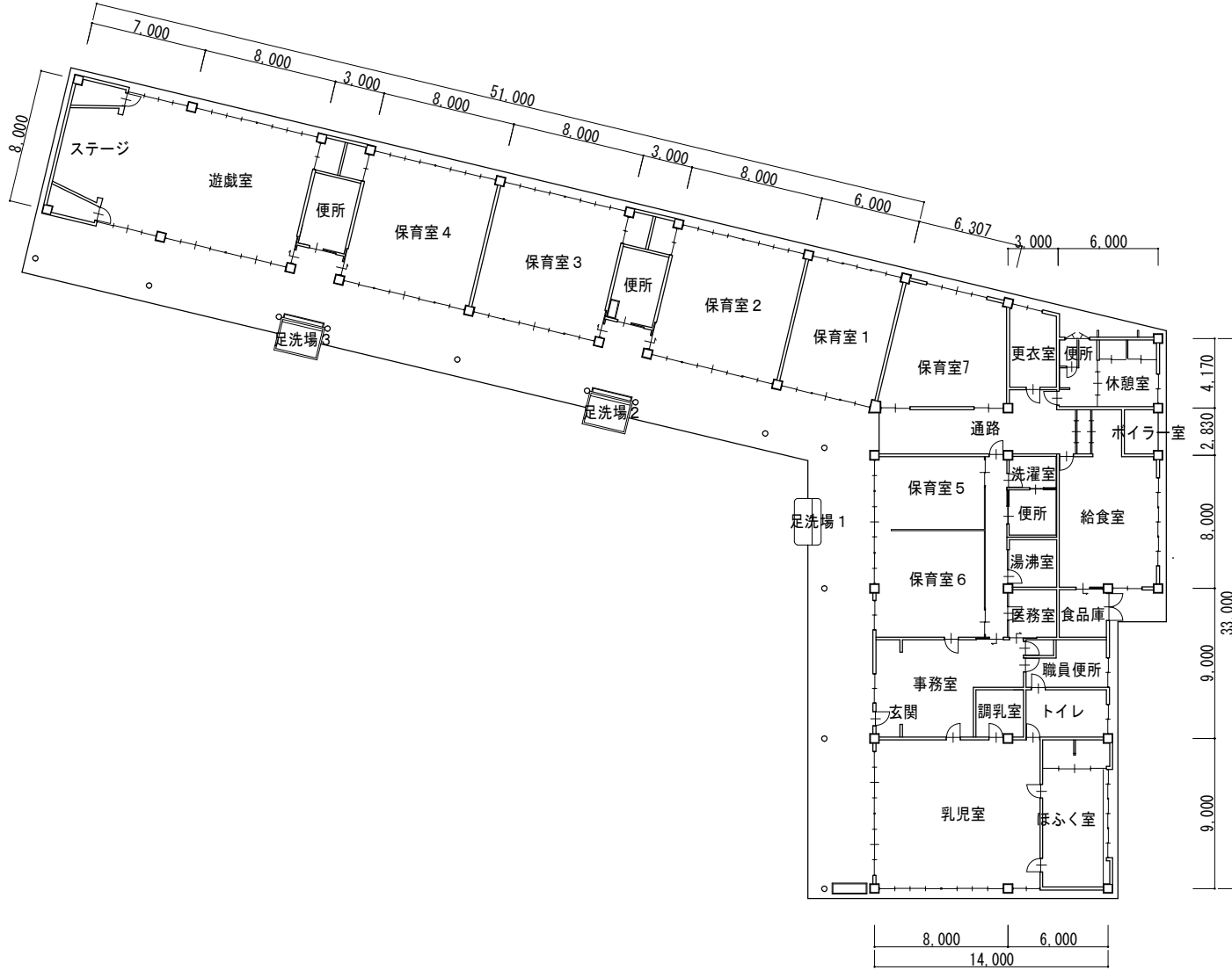
1 階 平 面 図
