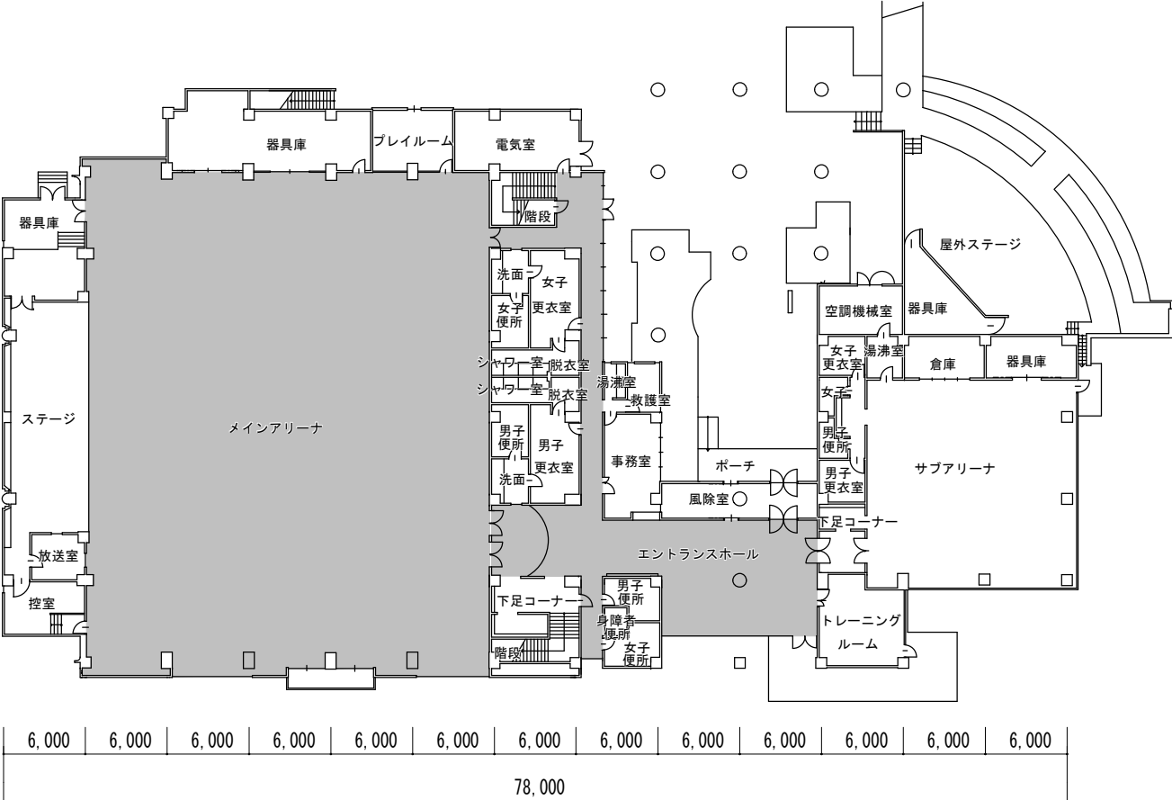
1階平面図
