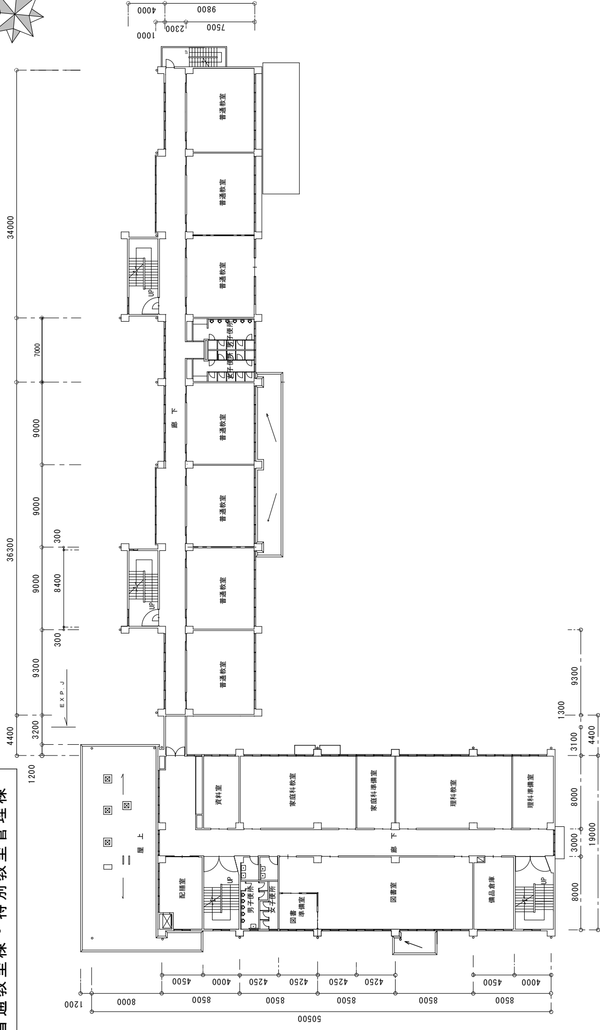
2階平面図
