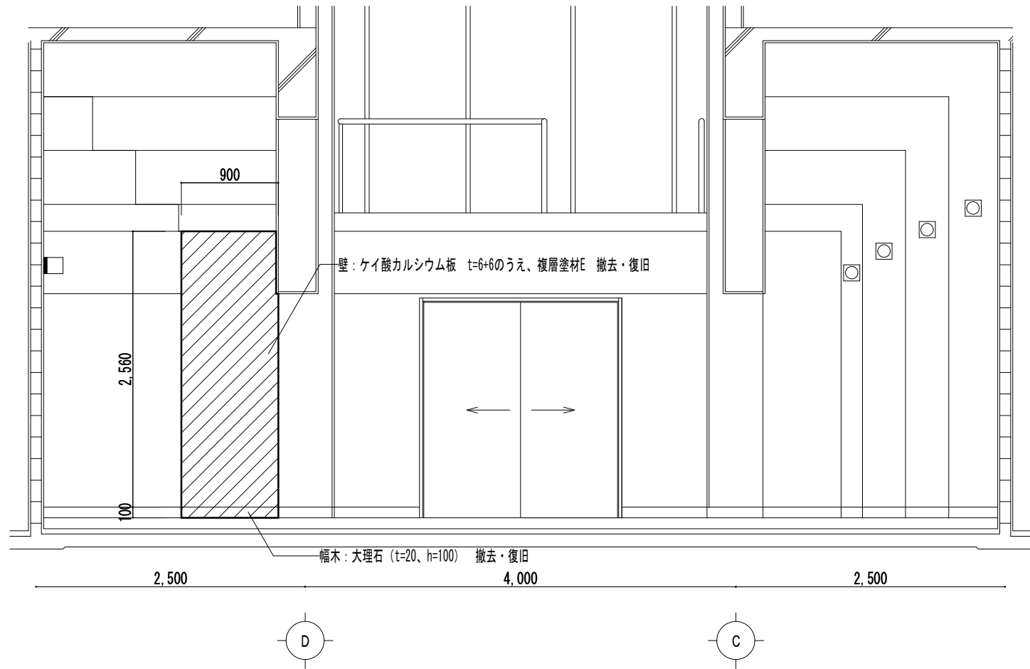
玄関ホール 展開図 S=1/50
