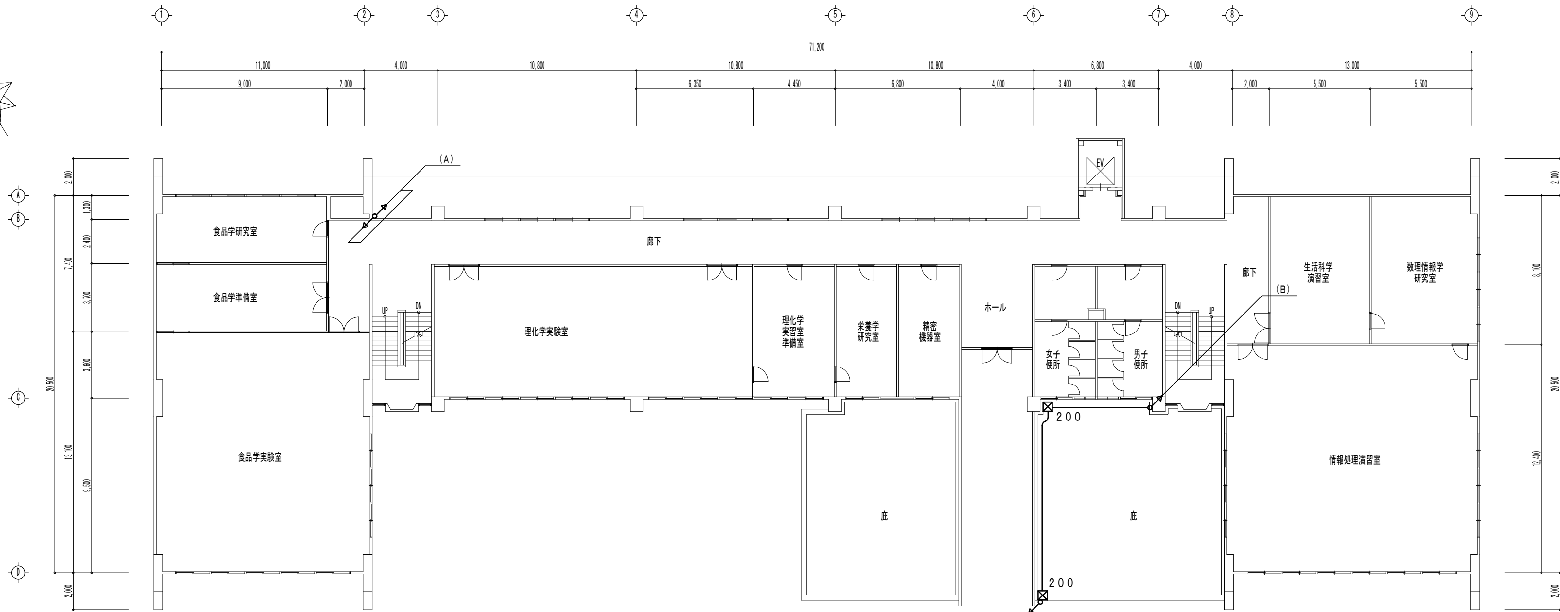
2階平面図 S = 1 / 200
