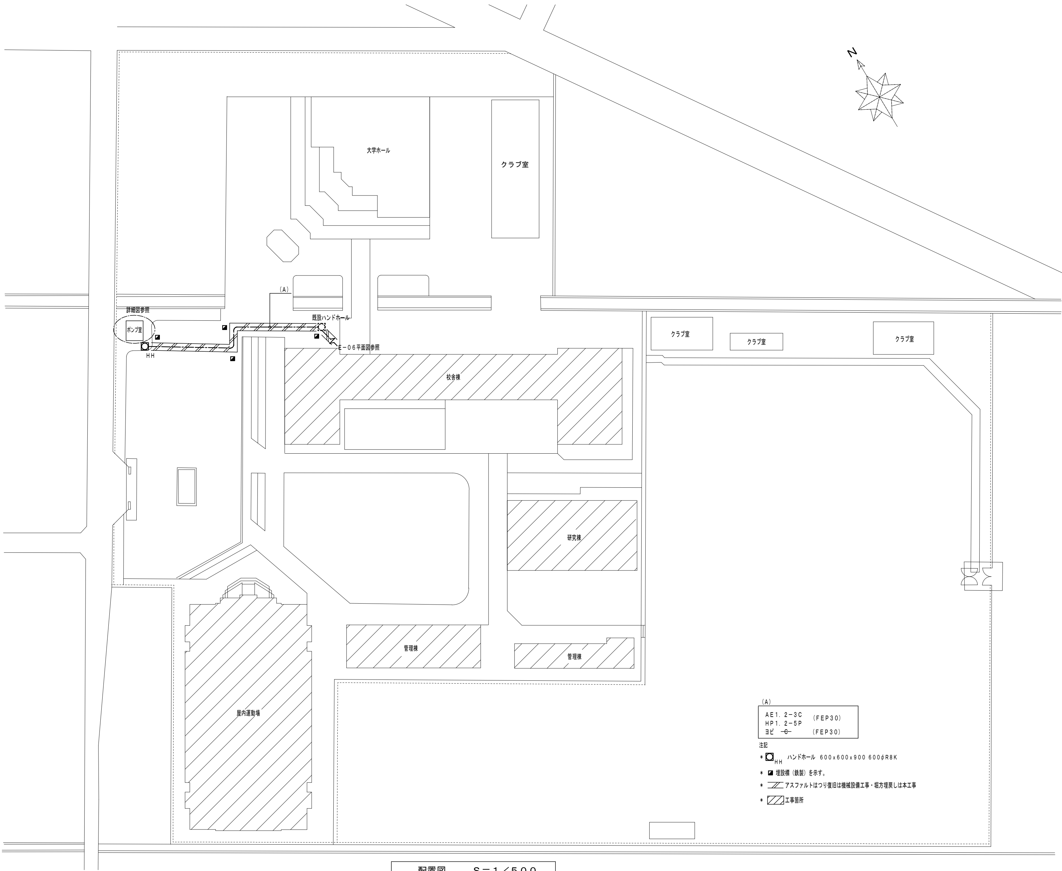
配置図 S = 1 / 5 0 0
