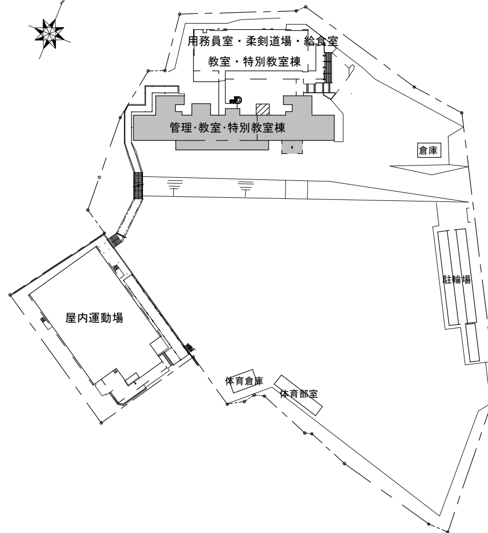
配置図
