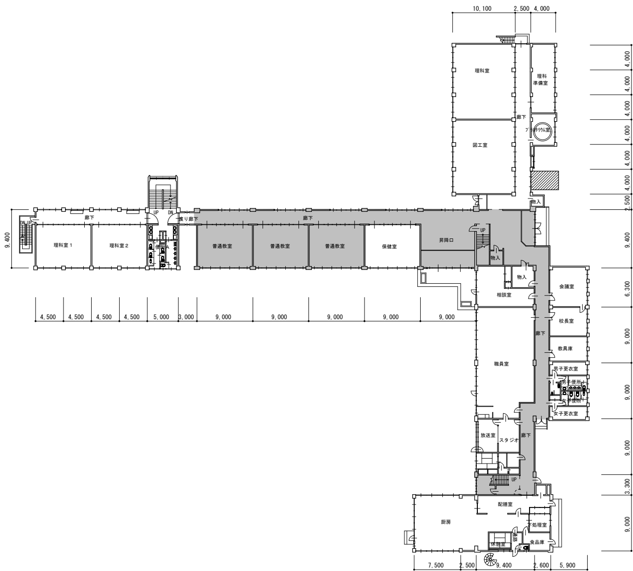
1 階平面図
