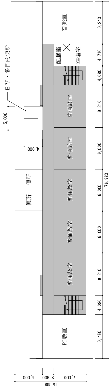
3 階平面図
