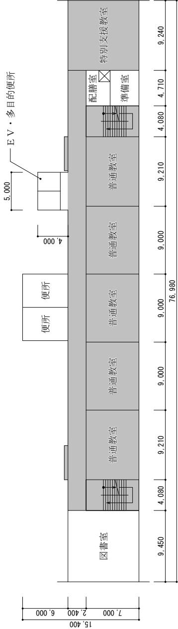
2 階平面図
