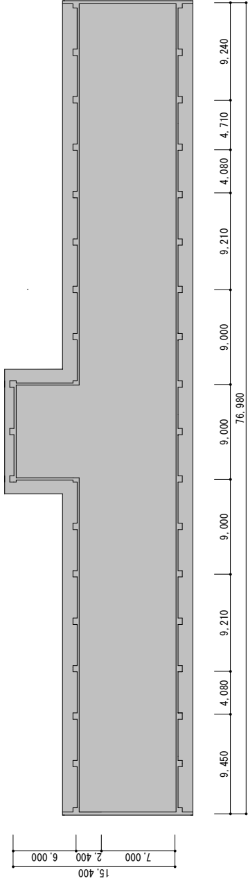
R 階平面図
