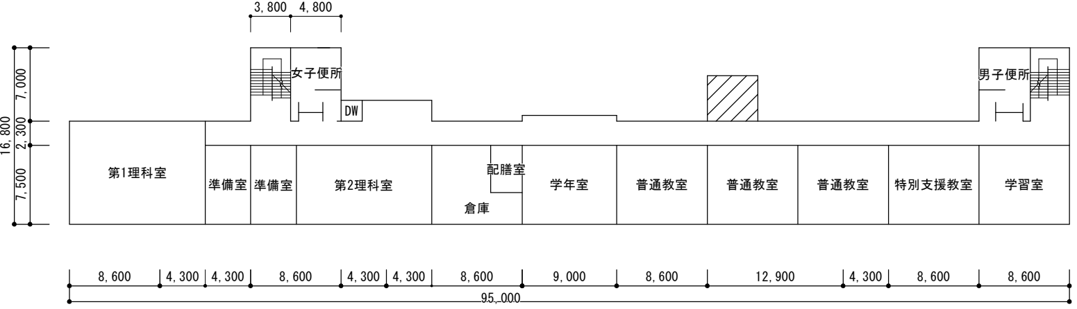
3 階平面図
