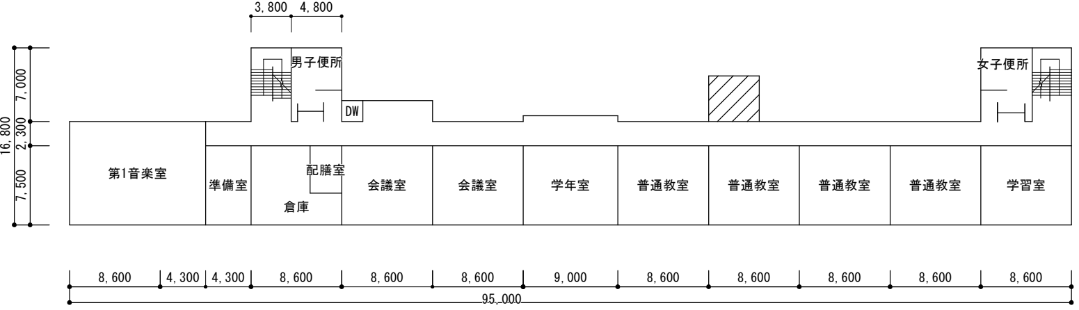
4 階平面図
