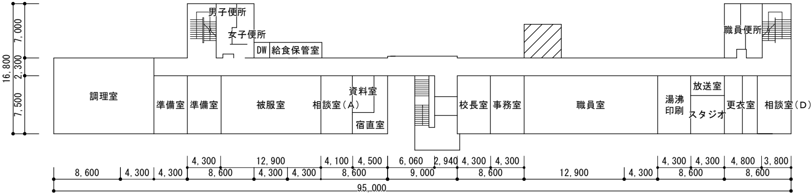
2階平面図
