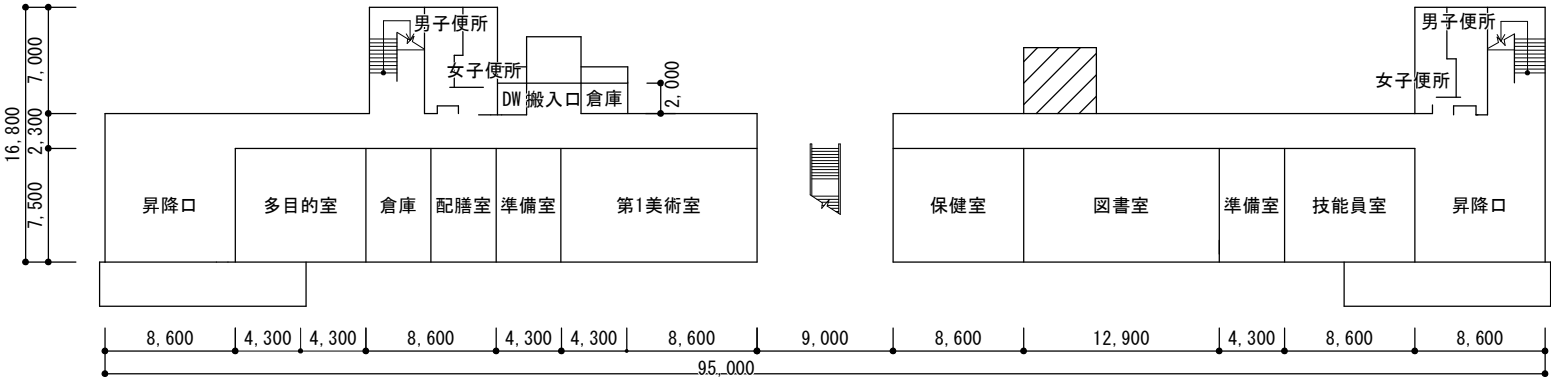
1階平面図
