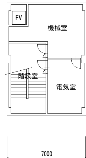
地階平面図
