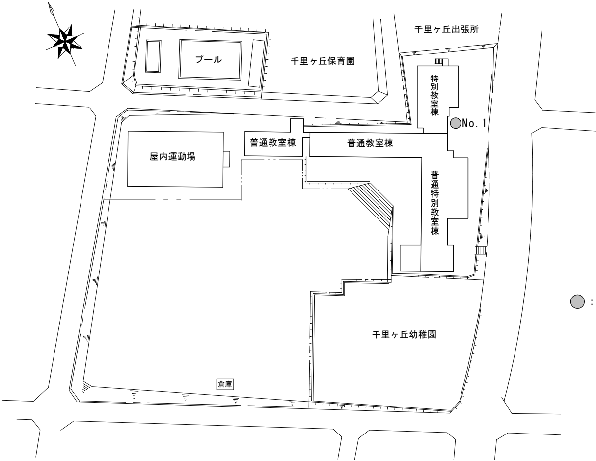
配置図
