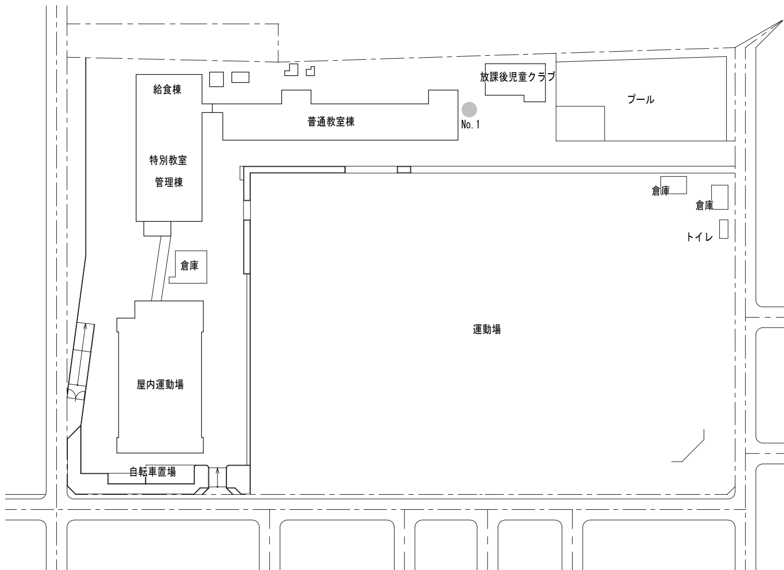
配置図
