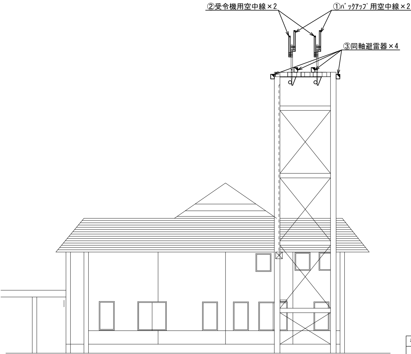
東立面図
