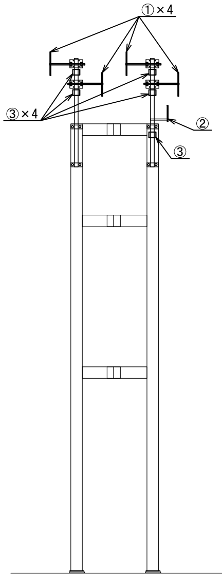
ホース乾燥塔
