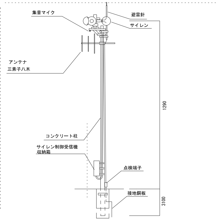
電柱設置例
