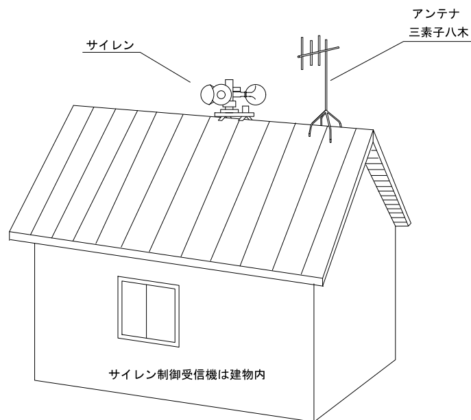
消防車庫設置例
