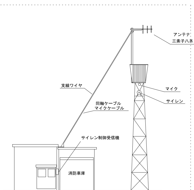
消防車庫・鉄塔設置例
