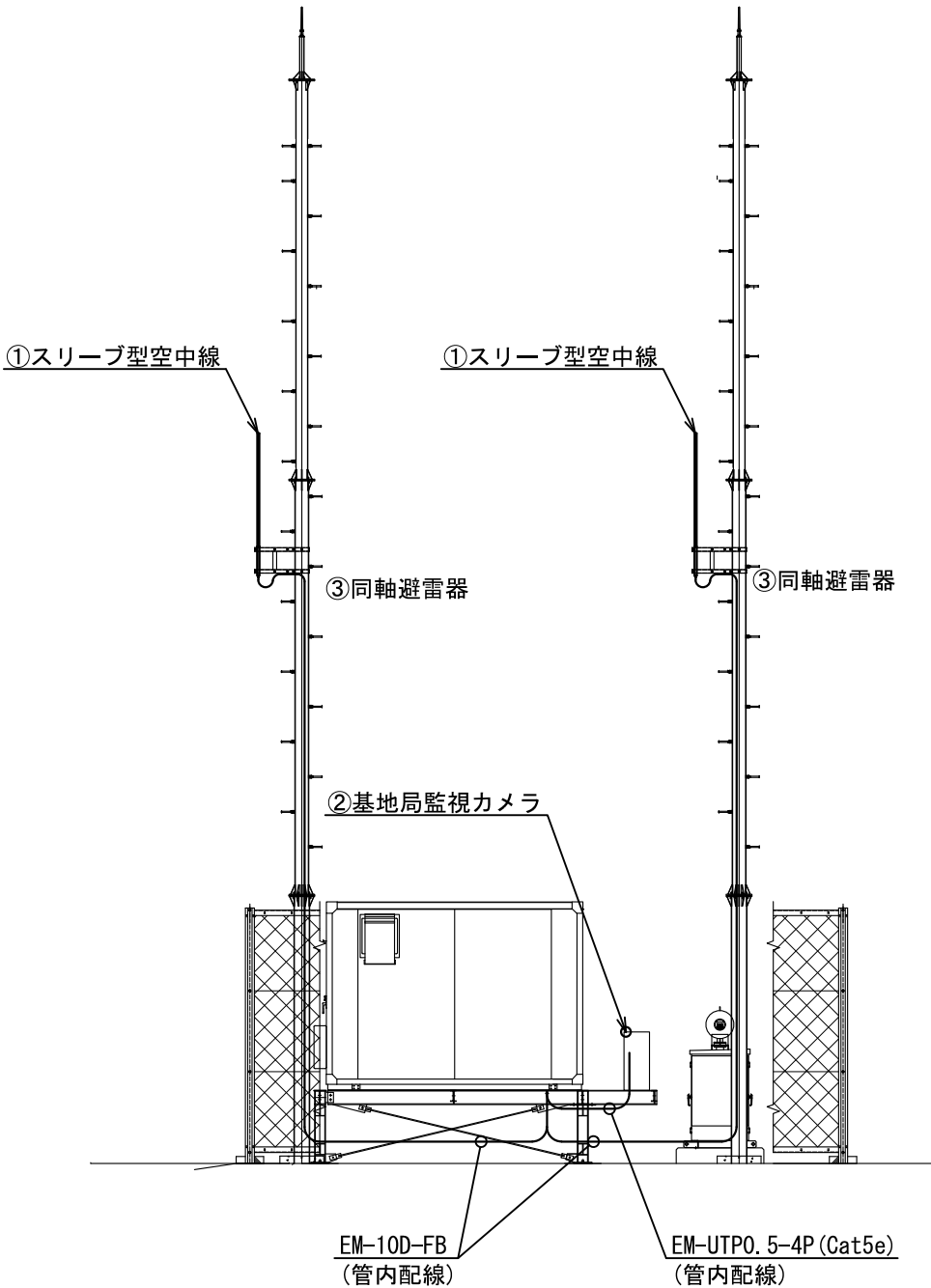
西立面図
