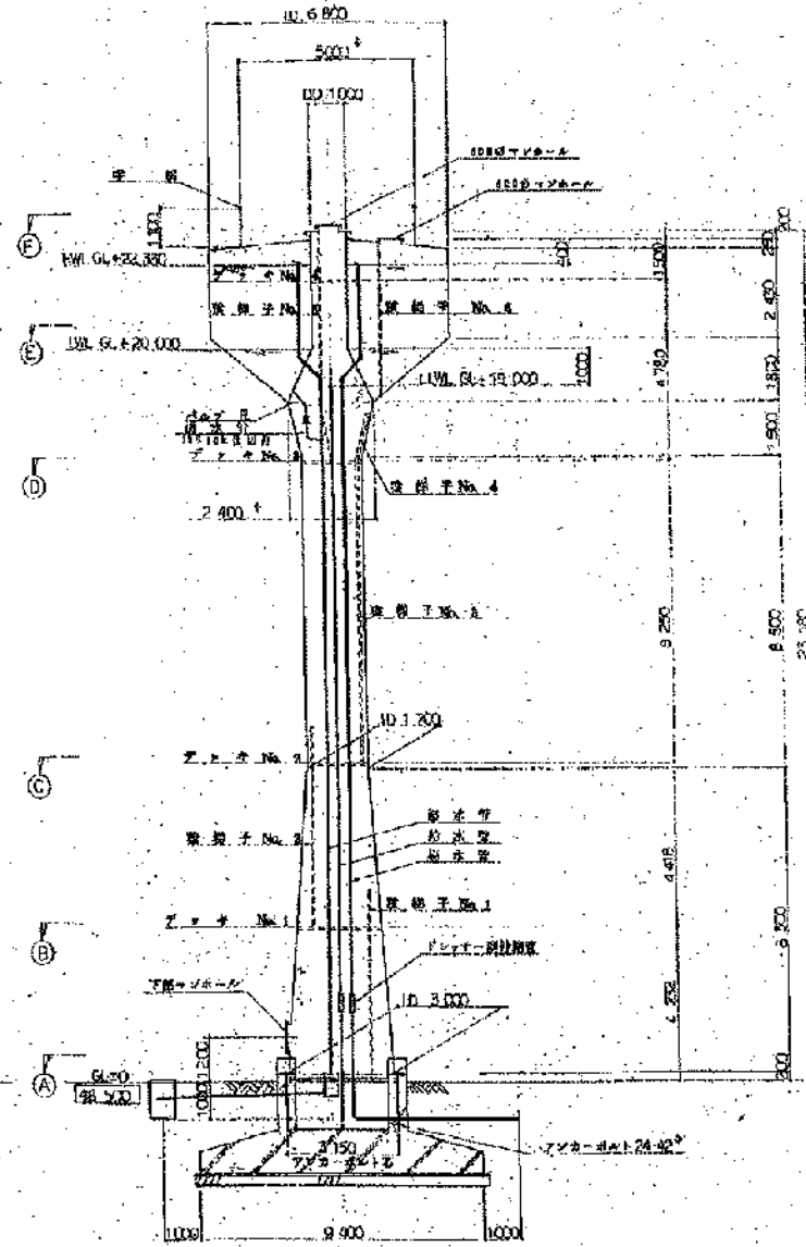
断面図
