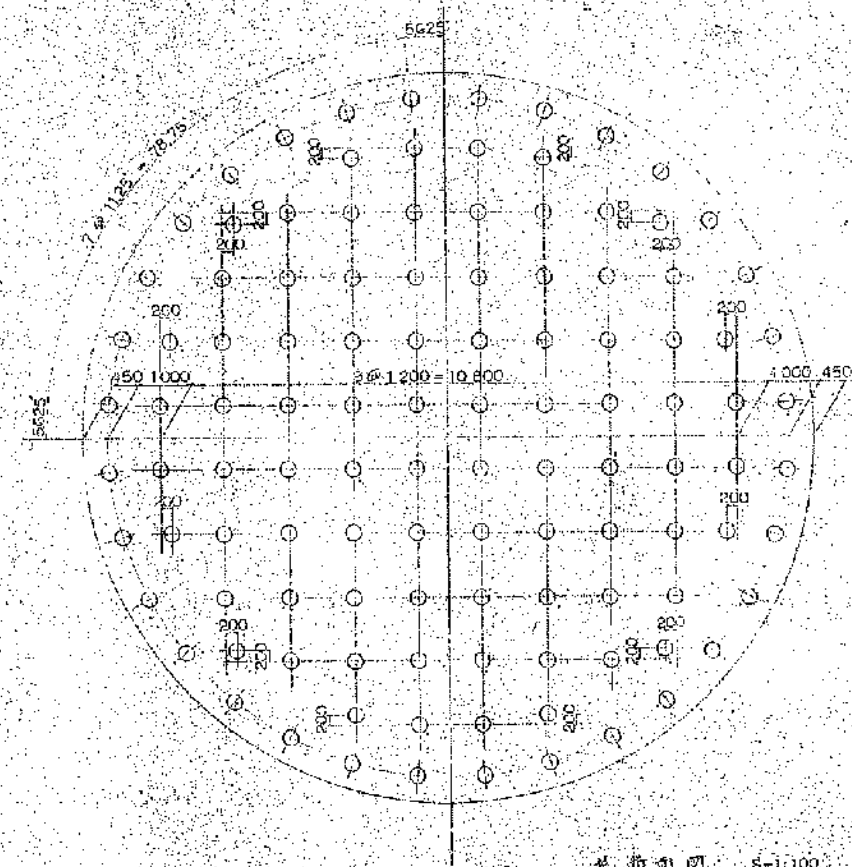
杭位図 S=1:100 (第1図、2図) 杭1本
