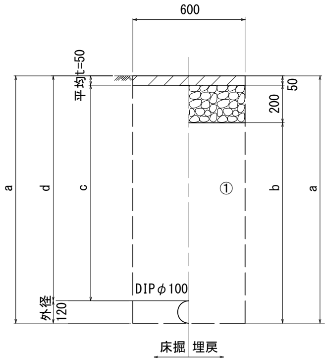
既設管撤去
