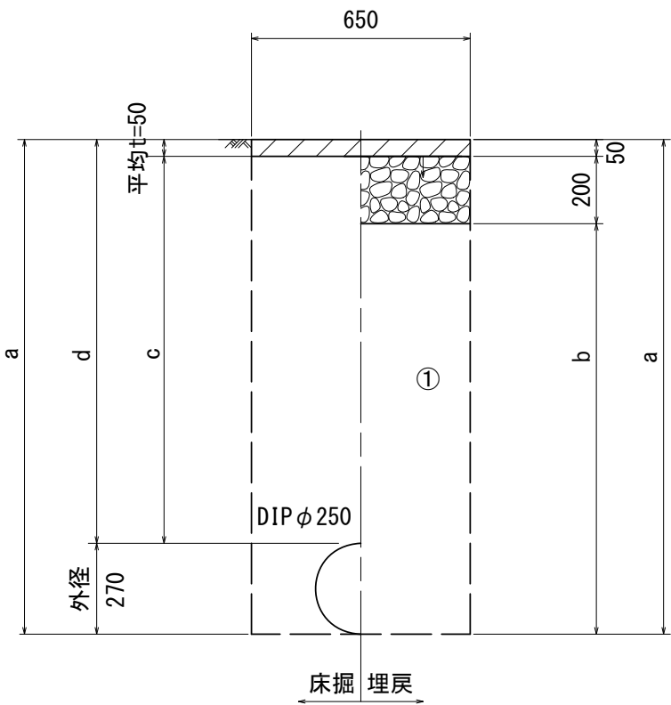
既設管撤去
