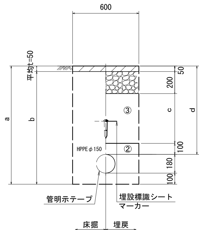
HPPE φ 150
