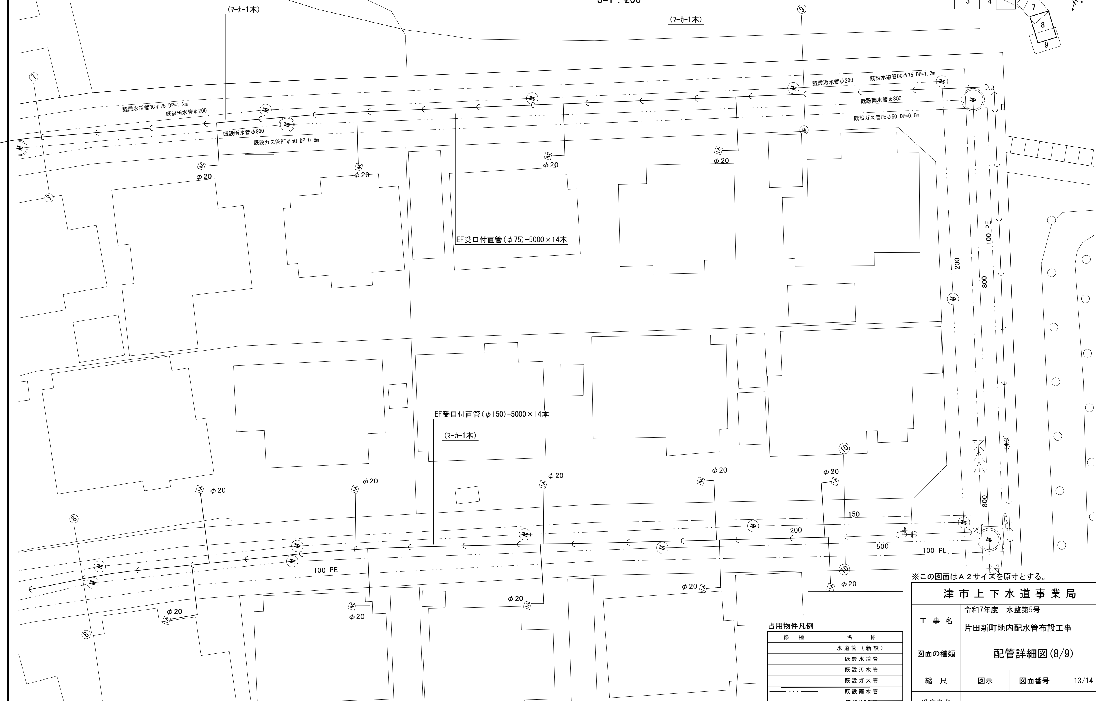
配管詳細図(8/9)
