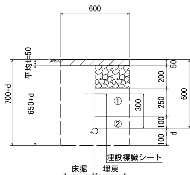
給水管
