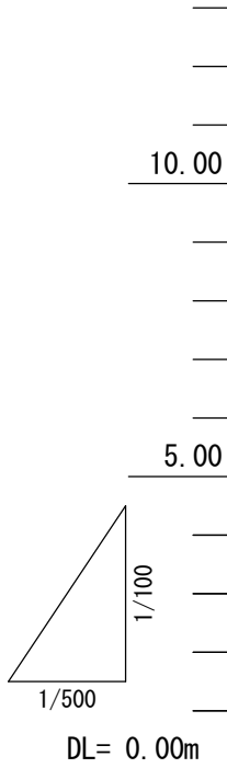
推進工縦断面図 V=1:100 H=1:500
