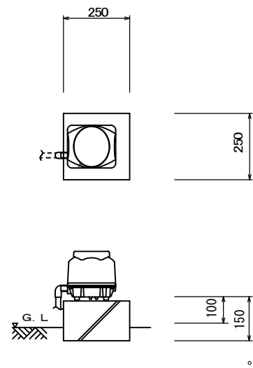
ブロー据付図 S=1/20
