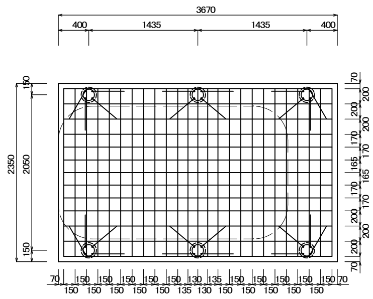
基 礎 配 筋 図 S=1/50
