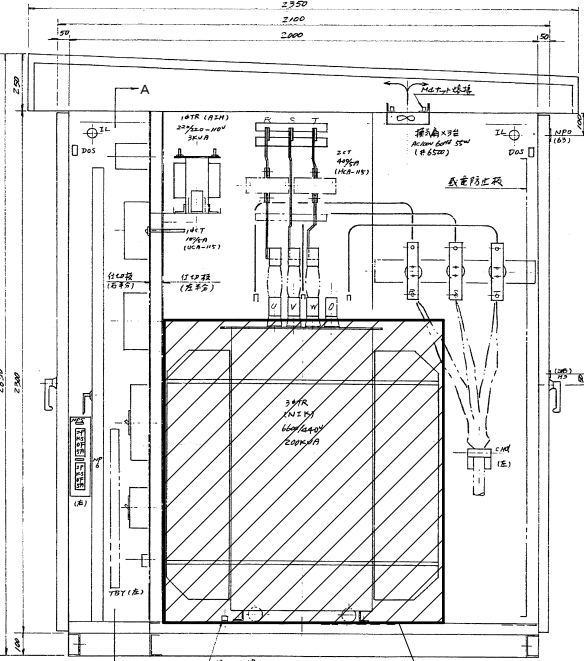
(側面図)
