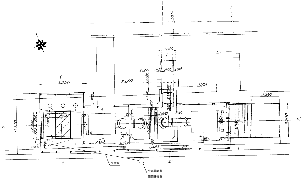
配置図
