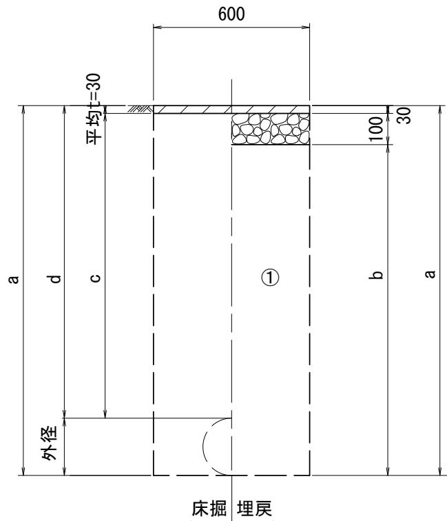
既設管撤去 県道歩道
