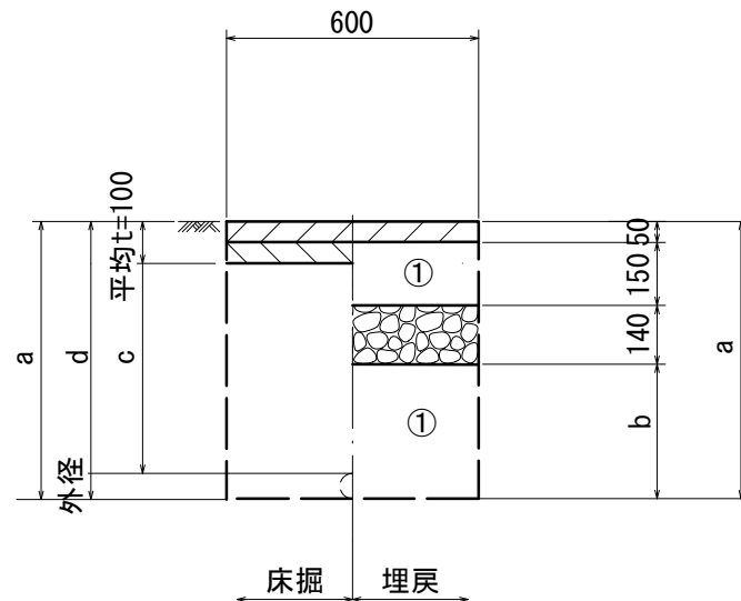
既設管撤去 県道車道舗装 (N5交通)
