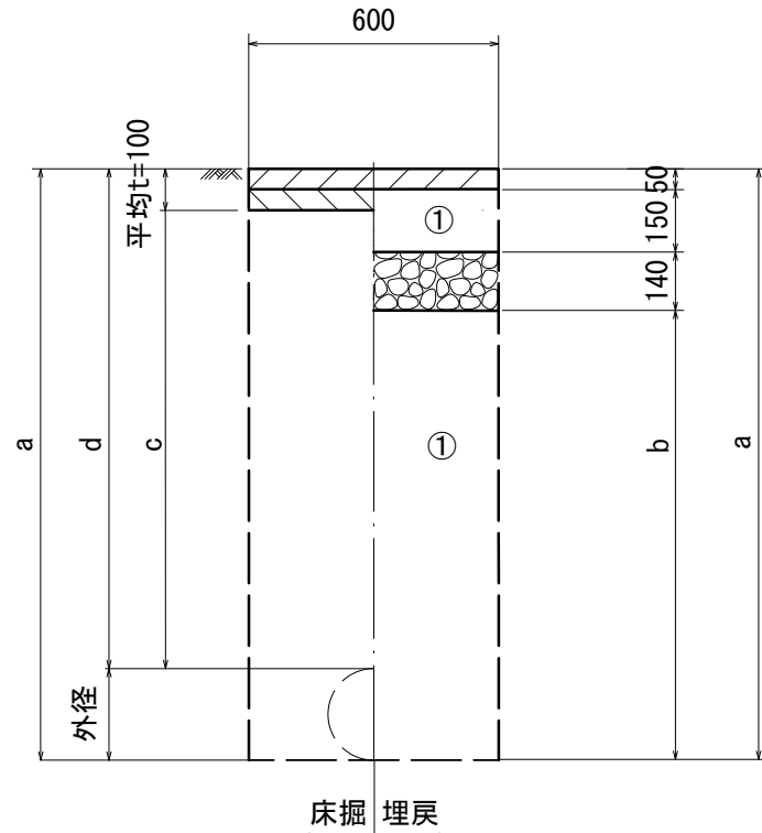
既設管撤去 県道車道舗装 (N5交通)
