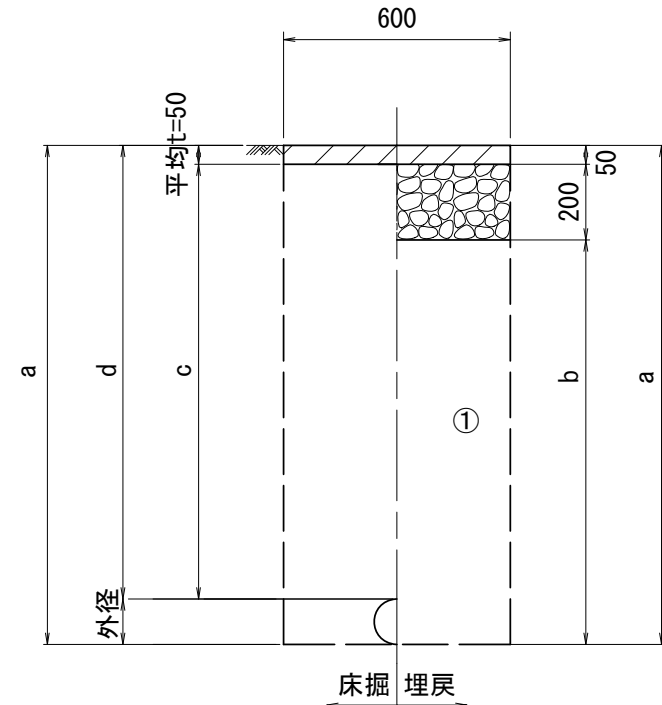
既設管撤去 市道
