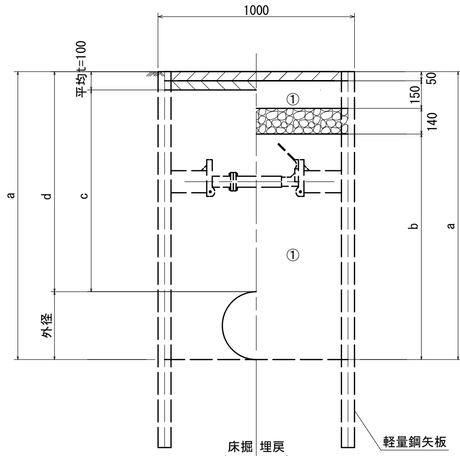
既設管撤去 県道車道舗装 (N5交通)
