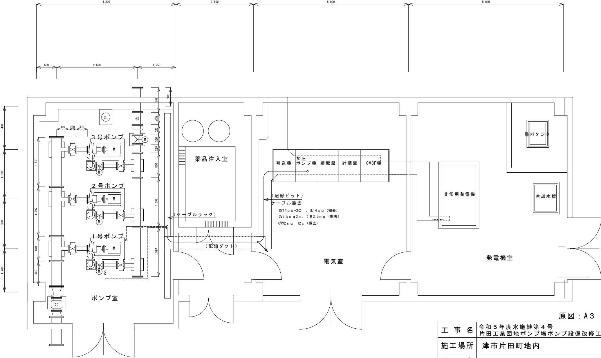
施設平面図（電線撤去範囲図）
