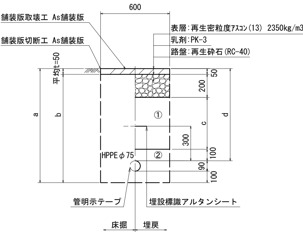
HPPEφ75 【市道部】
