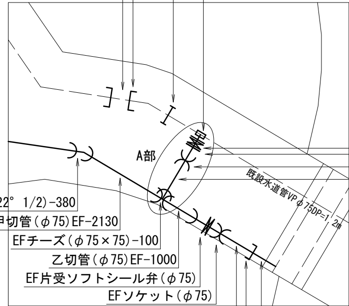
拡大図-1 S=1:100
