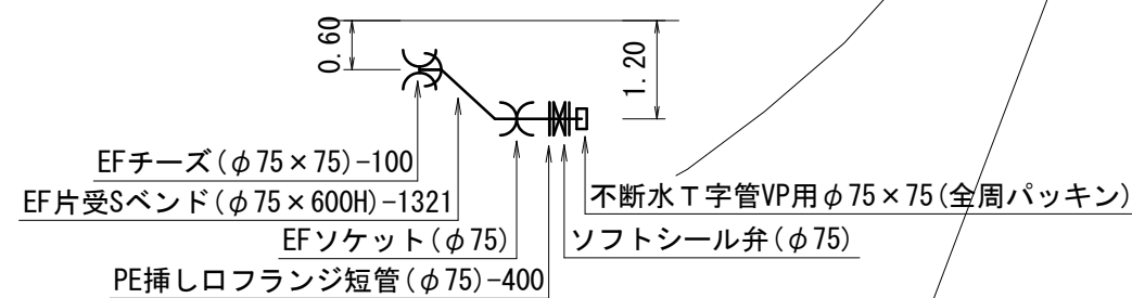
A部断面図 S=1:100
