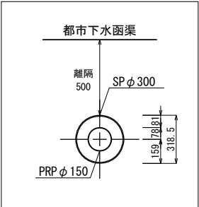
簡易推進部詳細図
