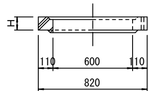
調整リング
