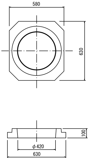
沈下防止板
