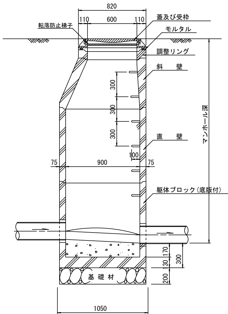
断面 A-A
