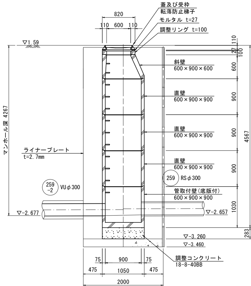
A-A断面図
