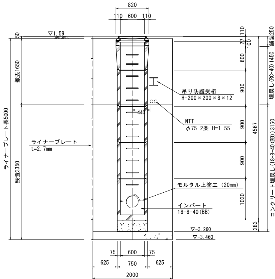
B-B断面図
