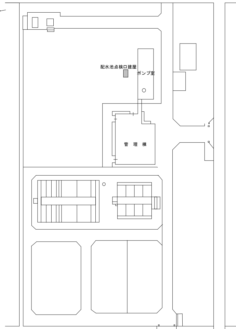
配置図
