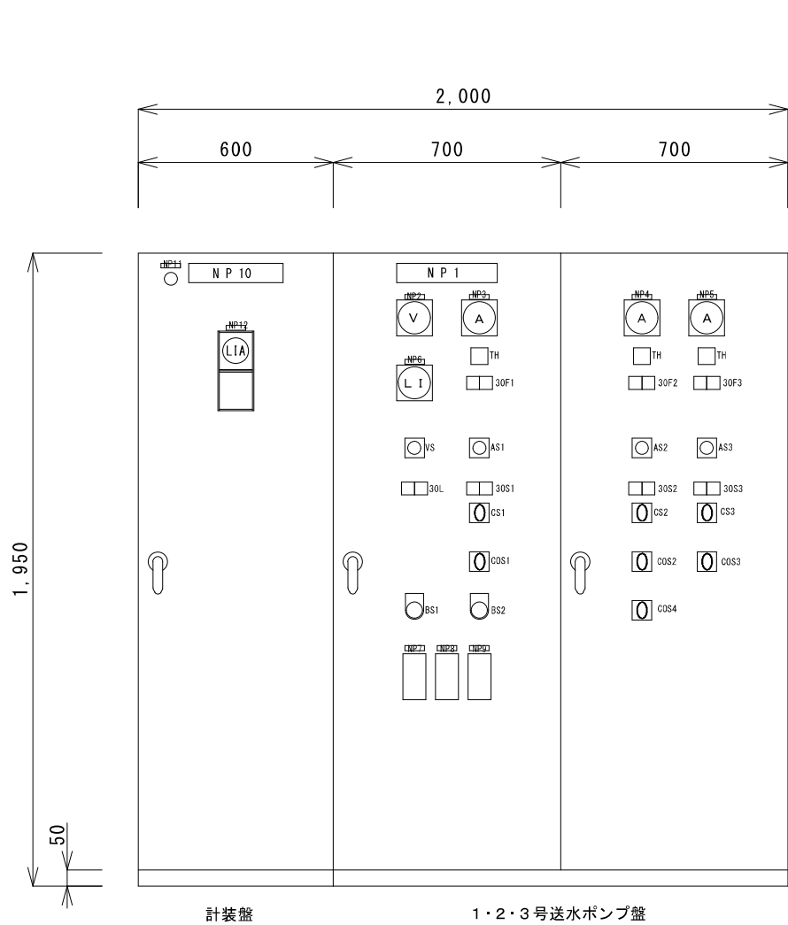
正面図 1/20
