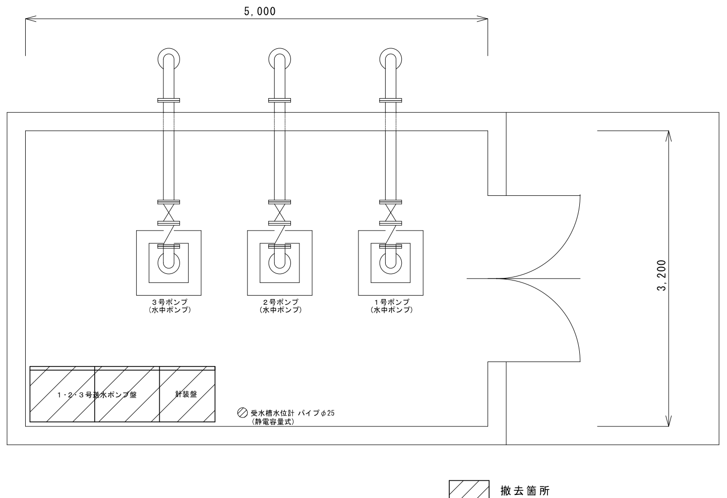
1・2・3号ポンプ室平面図 1/40
