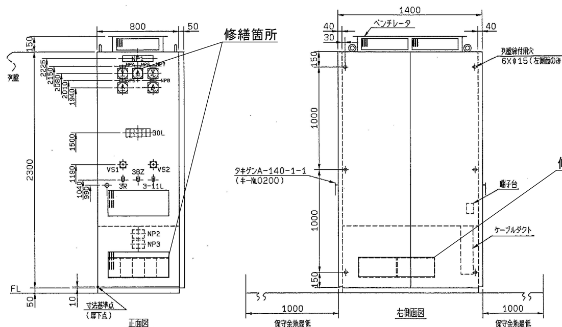
外形図
