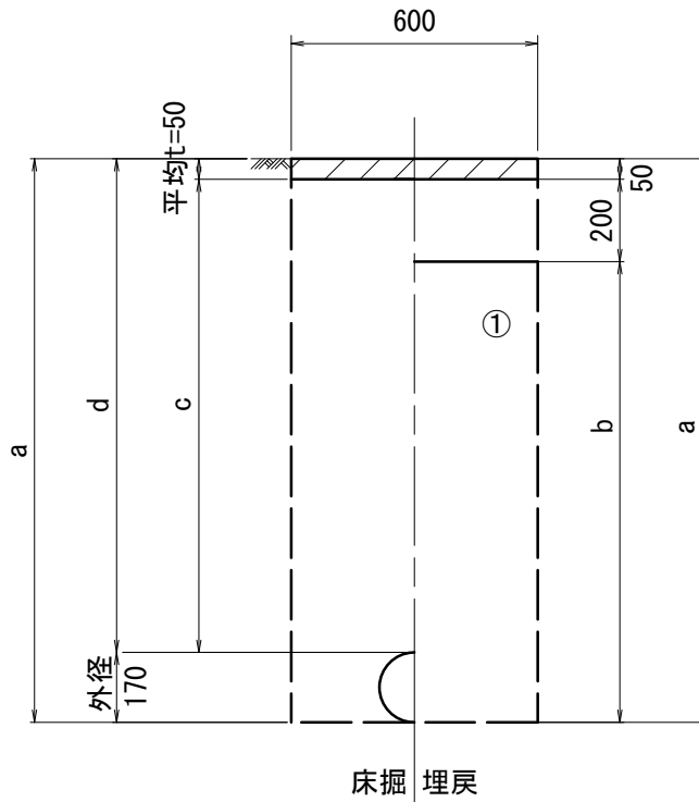
既設管撤去
