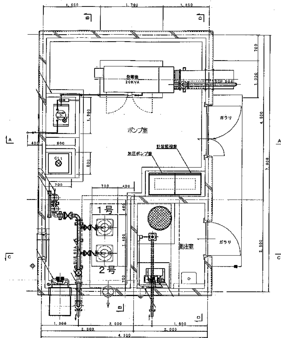
平面图
