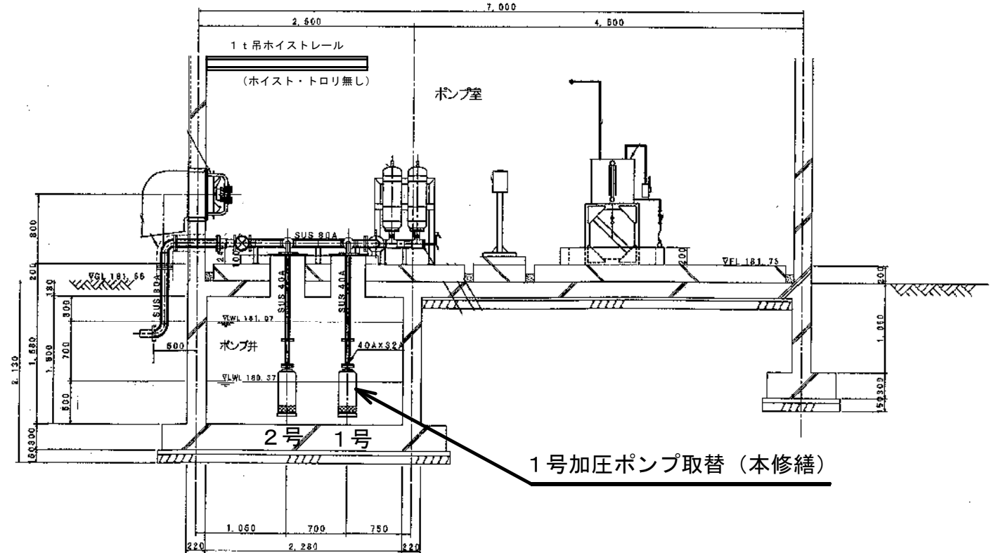
B—B 断面图
