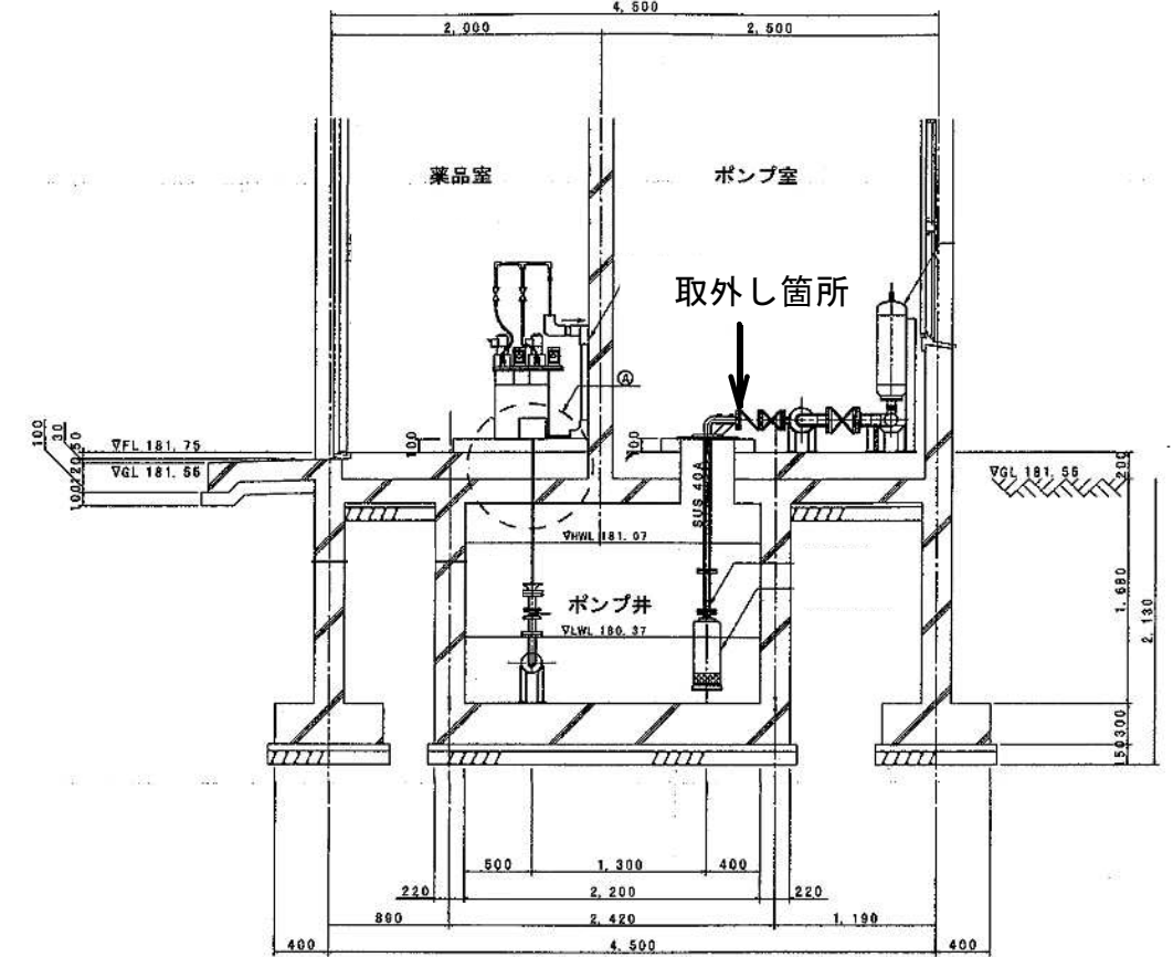
C—C 断面図
