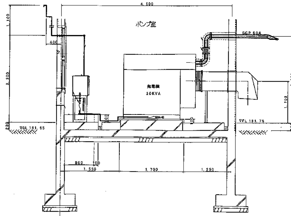
A — A 断面图
