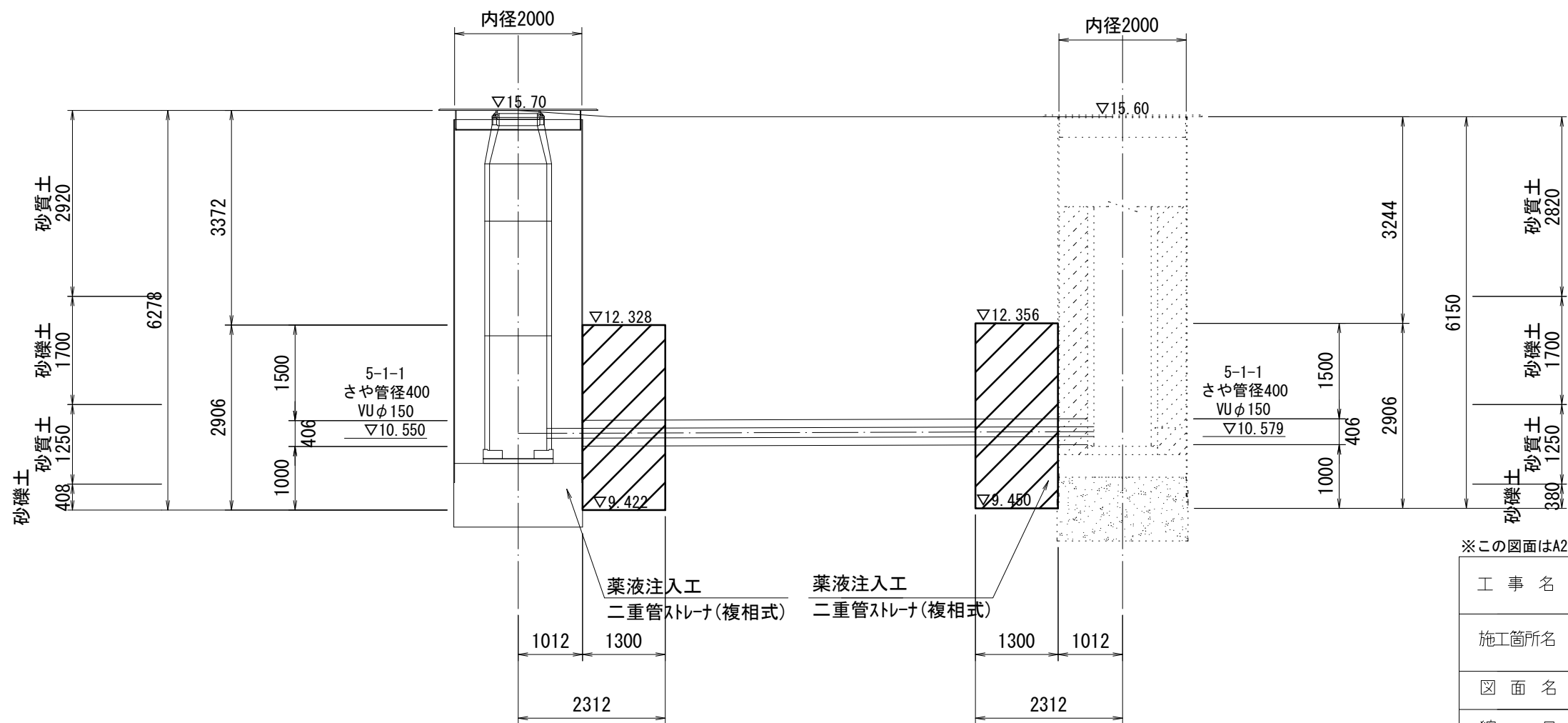
側面図
