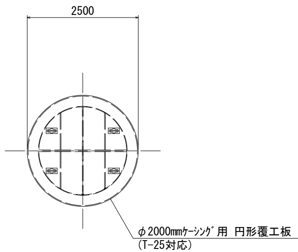
円形覆工板
