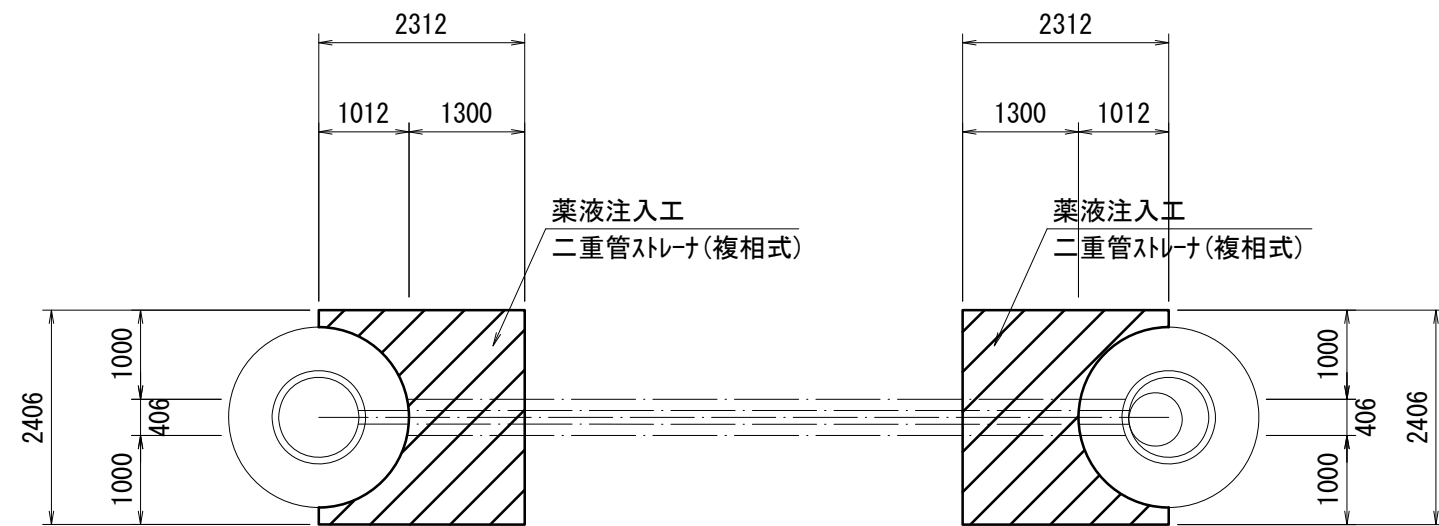
平面図
