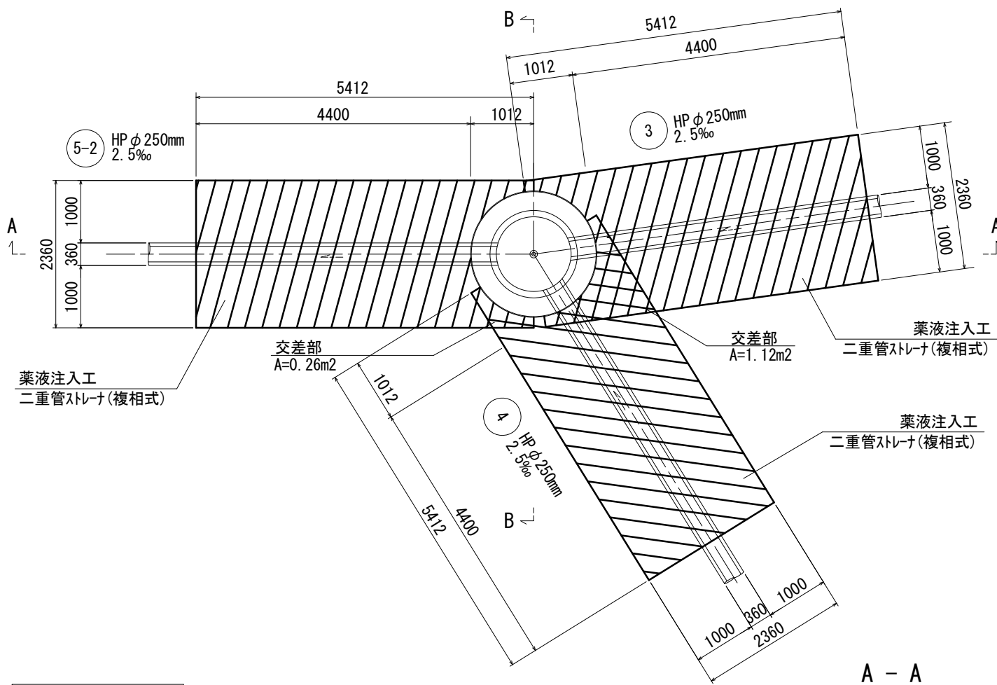
平面図
