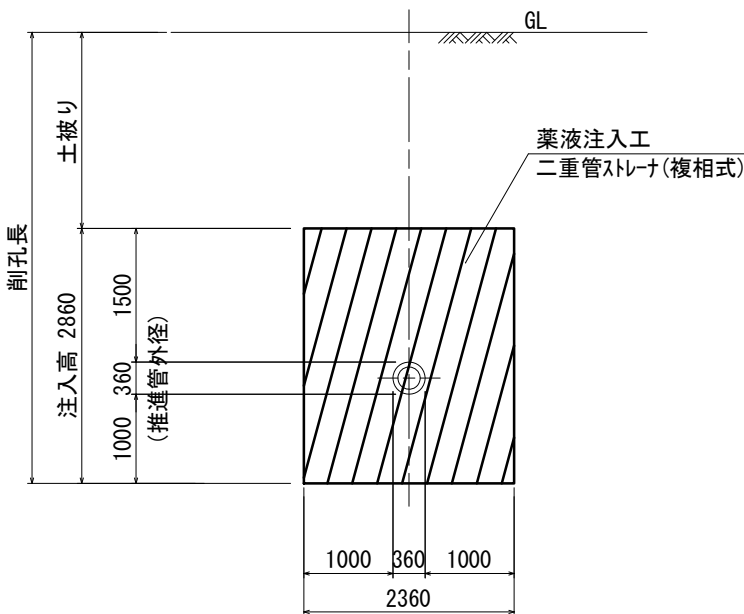
断面図
