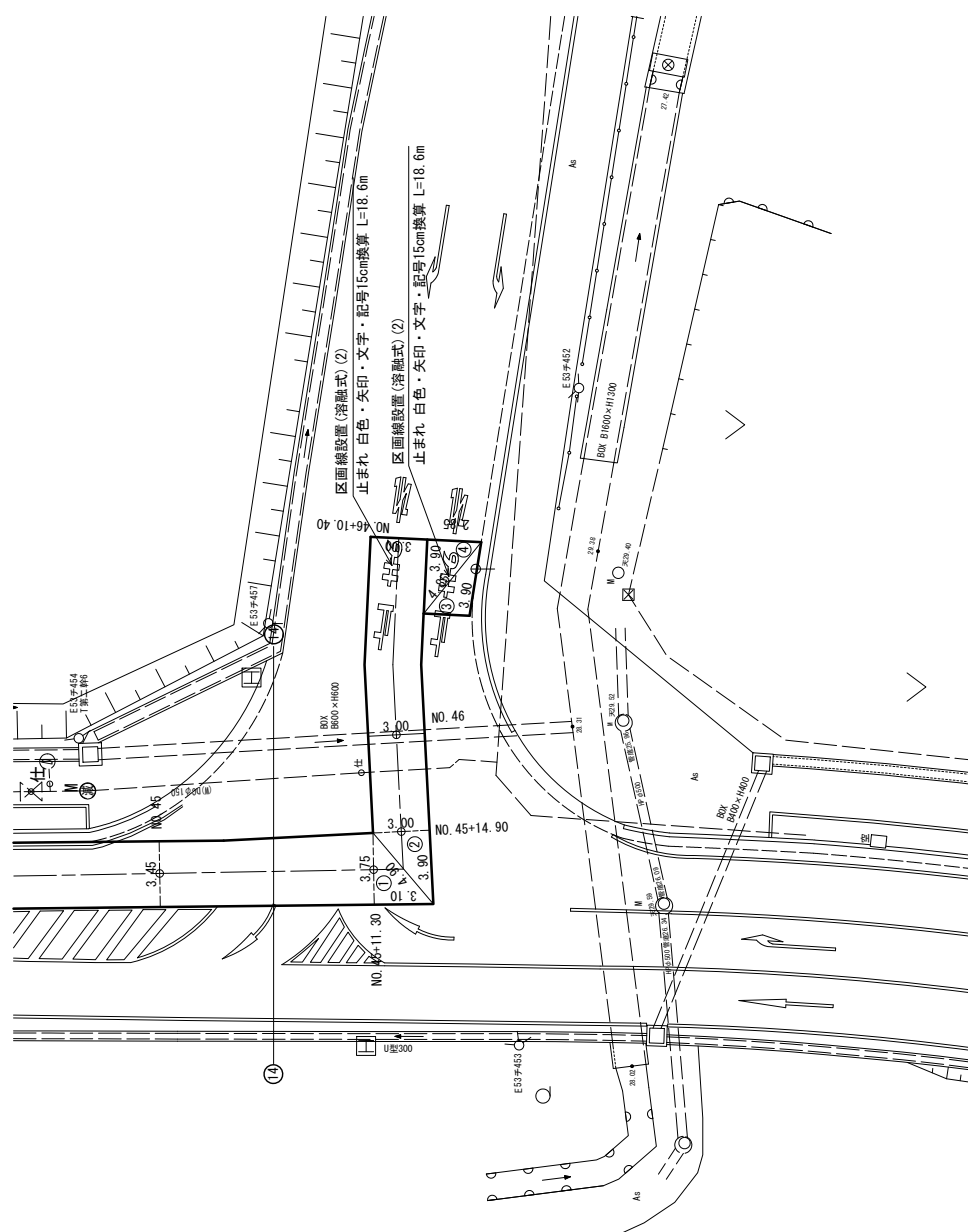
本復旧工平面図(14/14)
