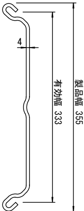
軽量鋼矢板 標準図 S=1/5
