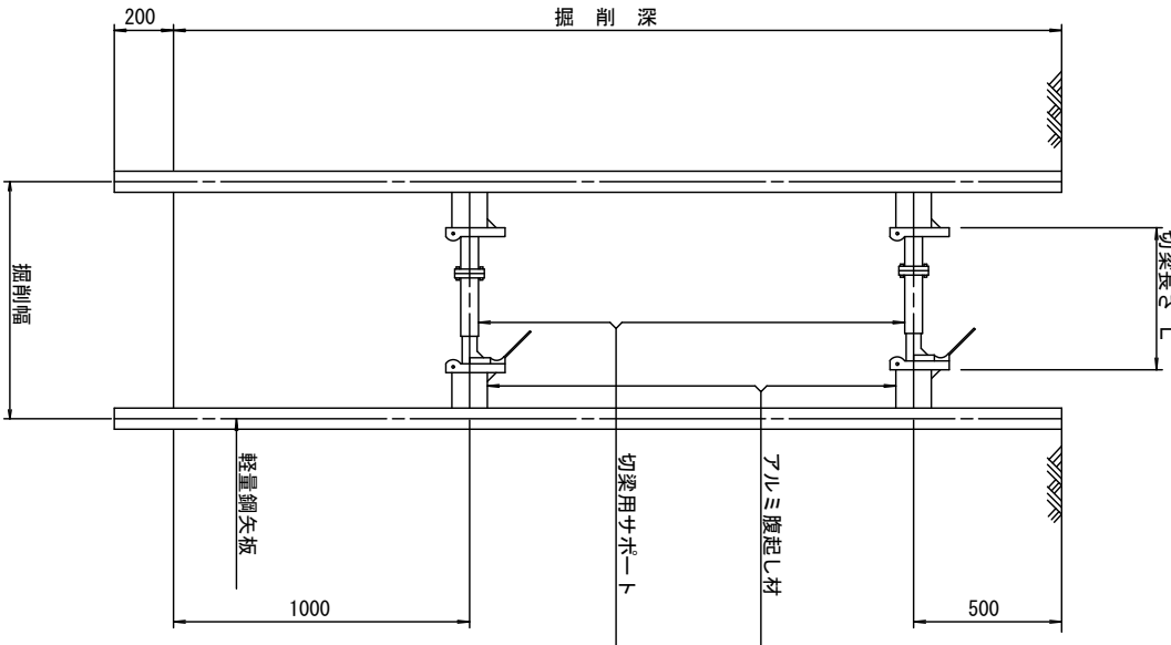
断面図 S=1/20
