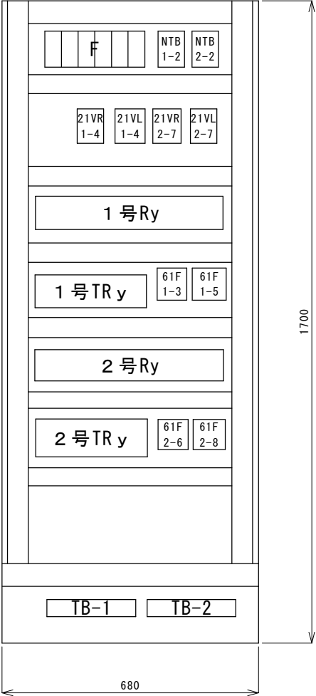
右側（既設）
