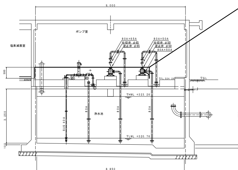
A-A断面図（今回更新工事後）
