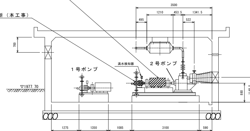
断面 B—B
