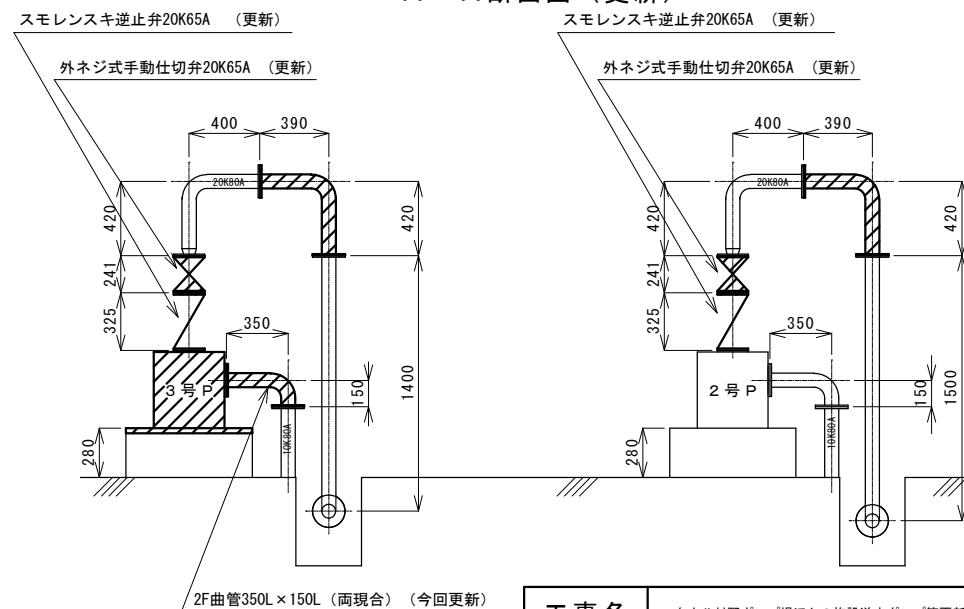
A—A 断面図（更新）
