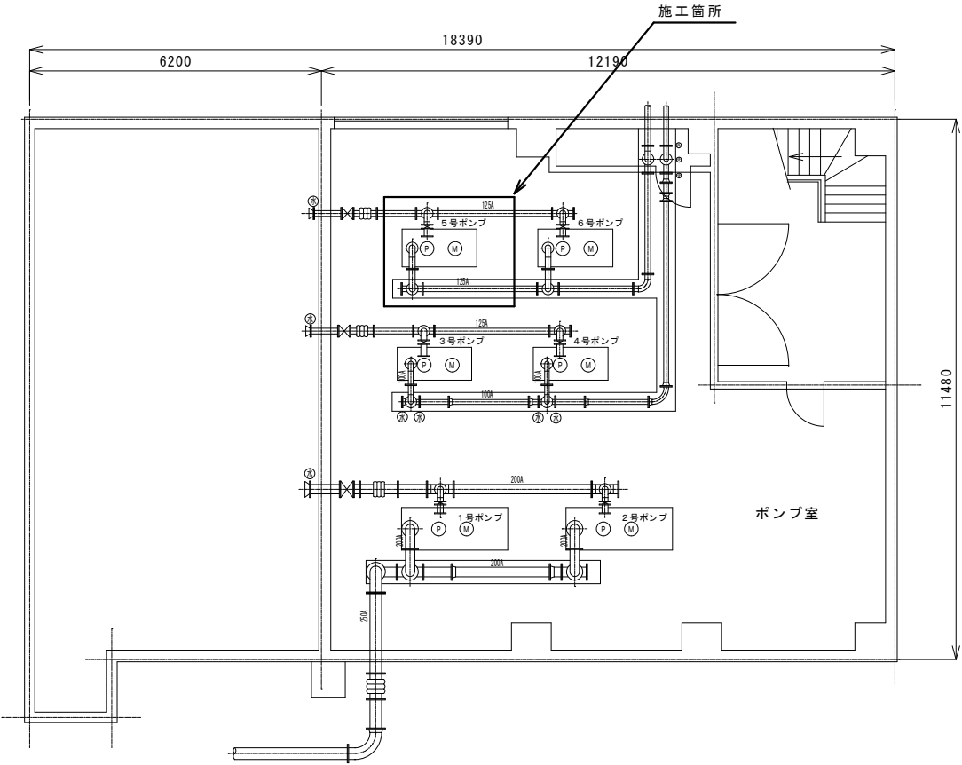
平面図
