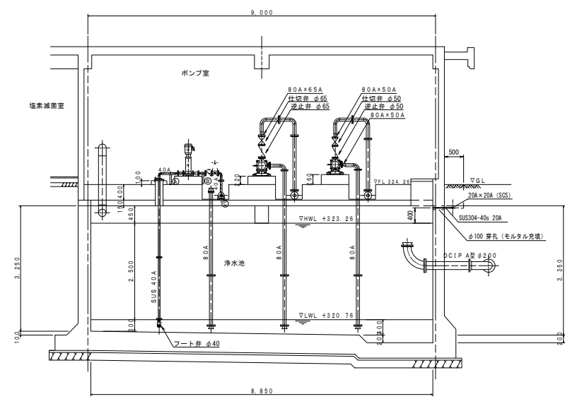
A-A断面図（既設）
