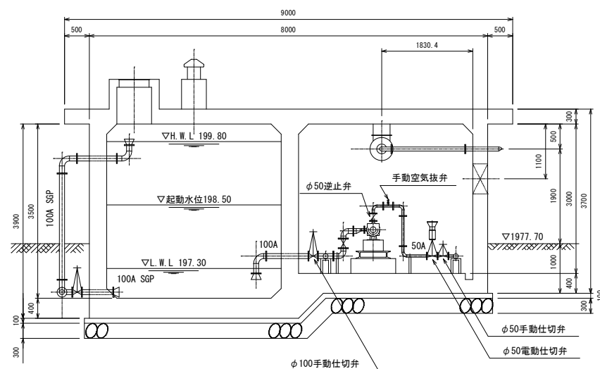
断面 A—A
