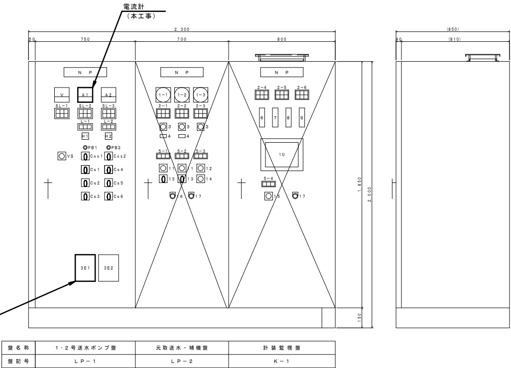
盤 姿 図
