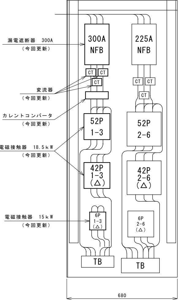
正面（今回更新後）
