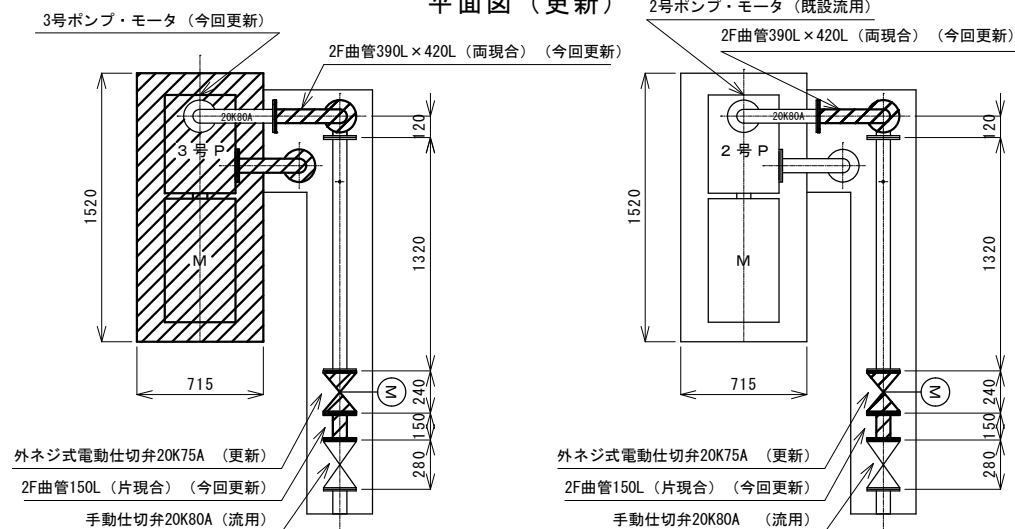
平面図（更新）
