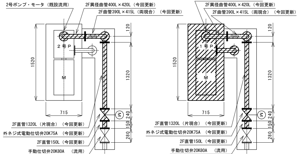
平面図（今回更新後）
