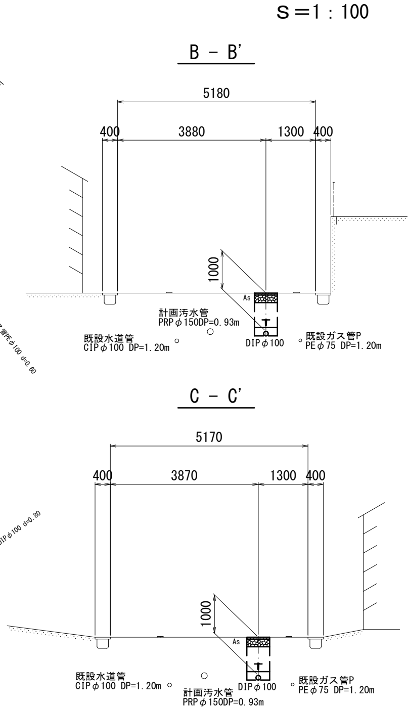
横断面図
