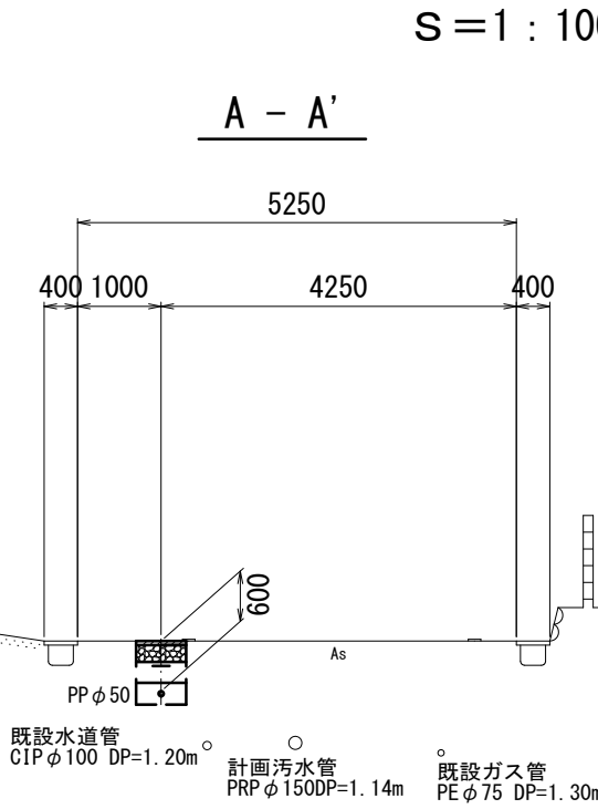
横断面図
