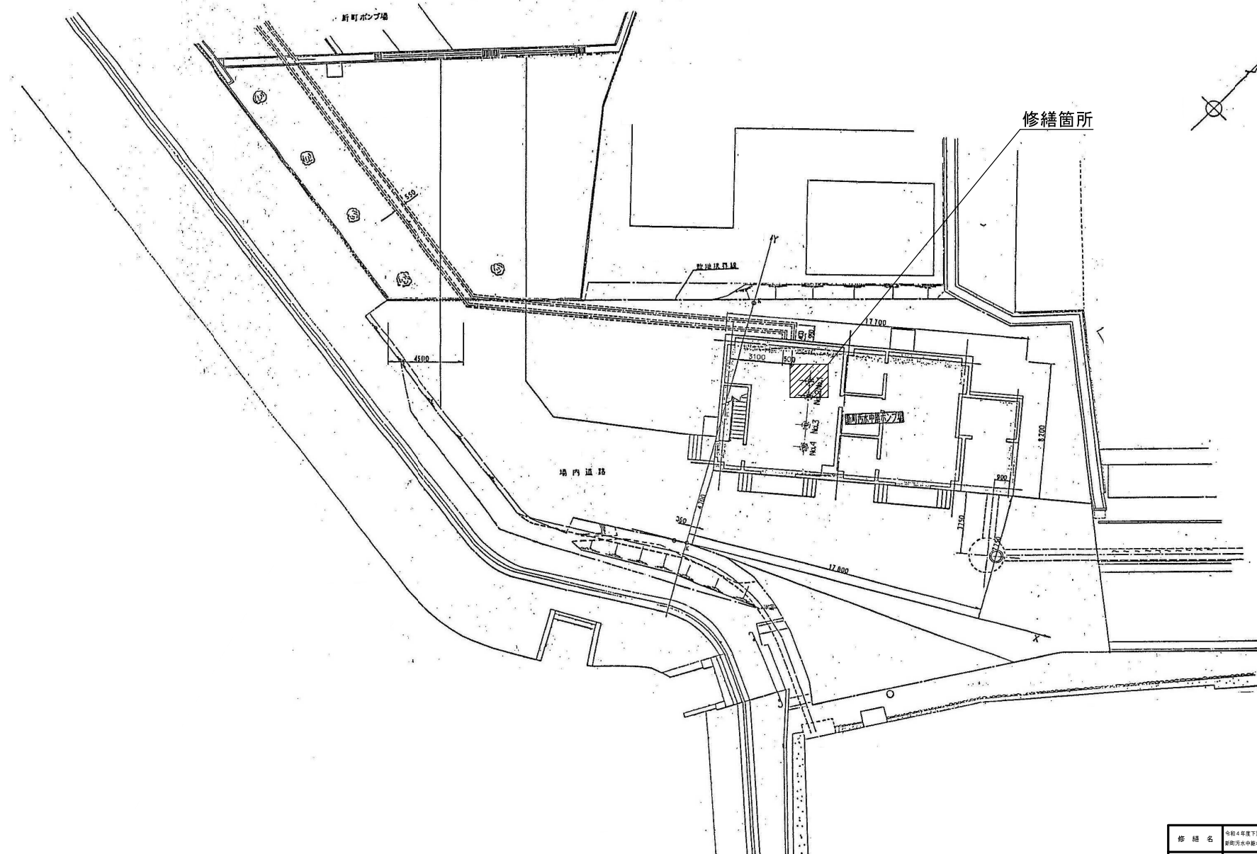
全体平面図
