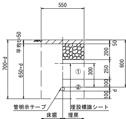
給水管
