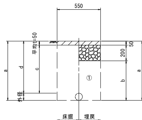
車道部 既設管撤去
