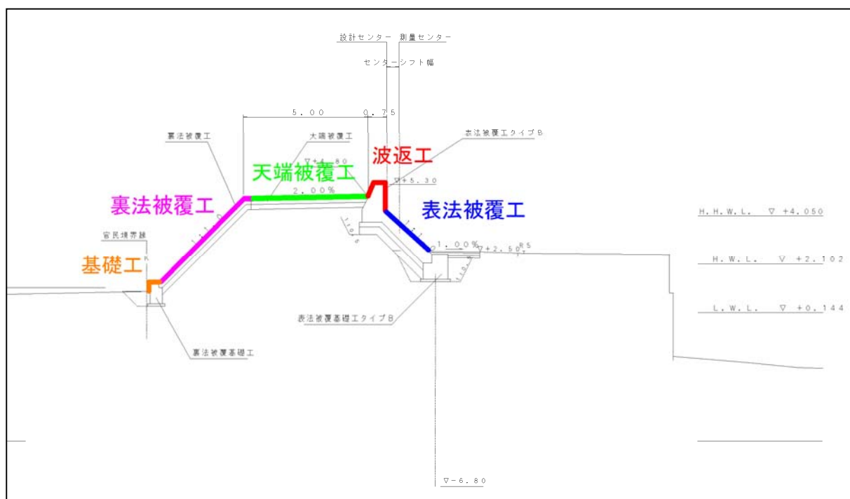
図 5-4 防汐堤③ 修繕費想定箇所
