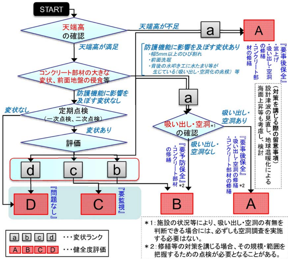
図 3-1 健全度評価のフロー
