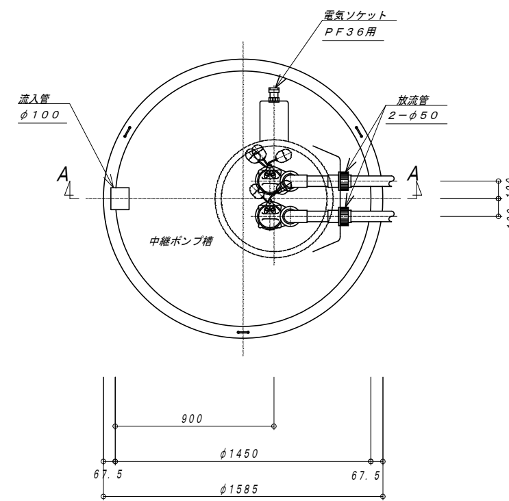
平面図 1:20
