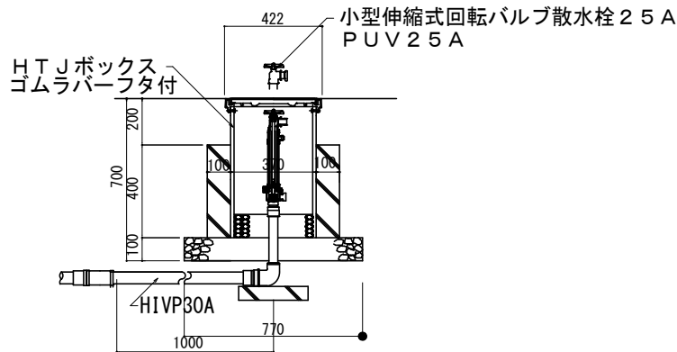
伸縮回転式小型散水栓 25A 詳細図 1:20
