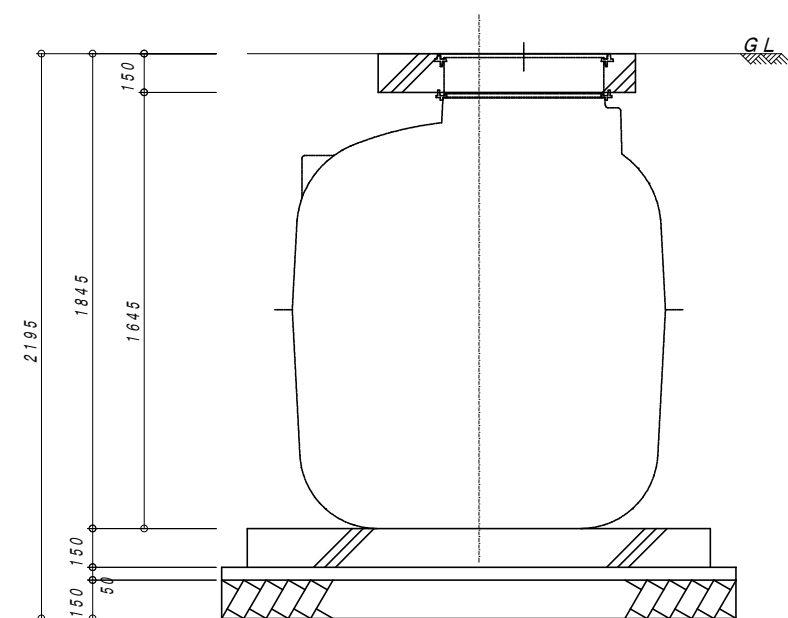
A-A 断面図 1:20
