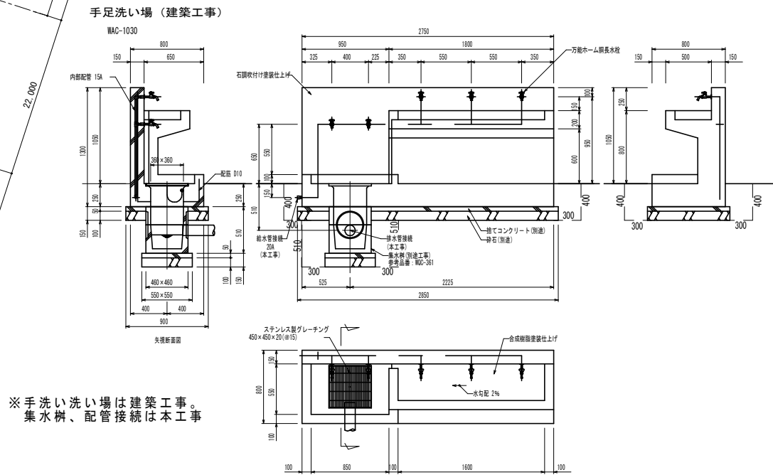
手足洗い場詳細図 1:40
