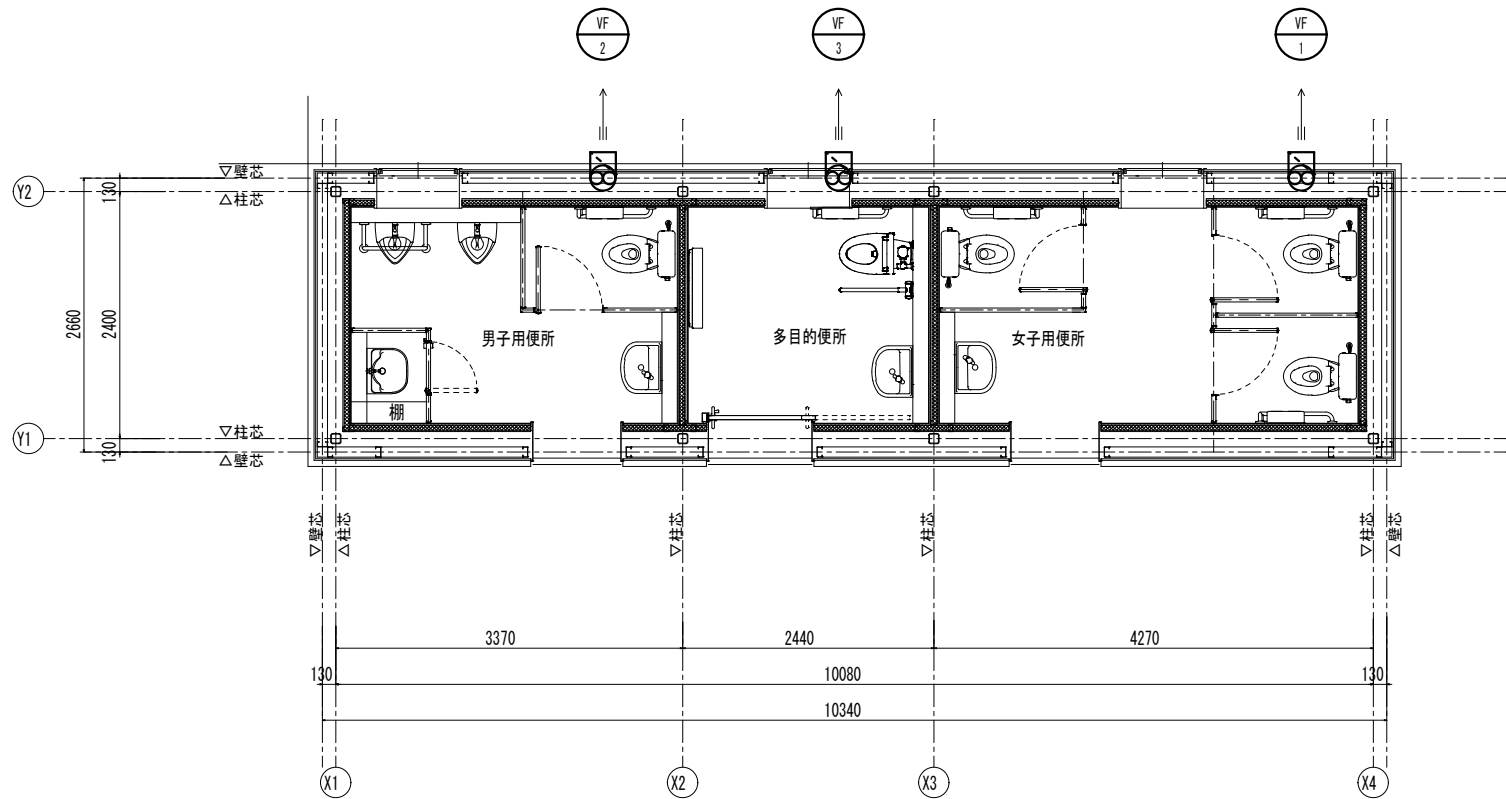
換気平面図 1/50
