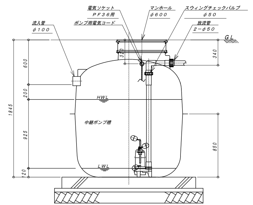
A-A 断面図 1:20
