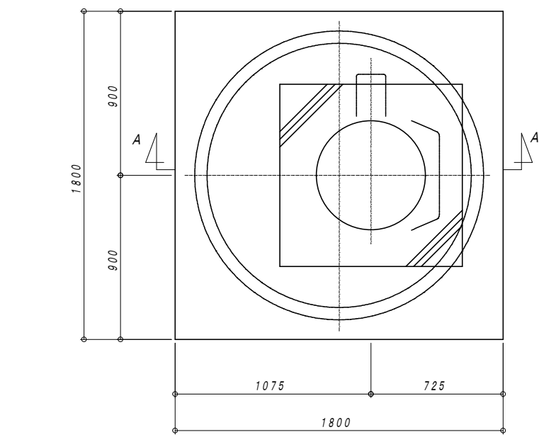
平面図 1:20
