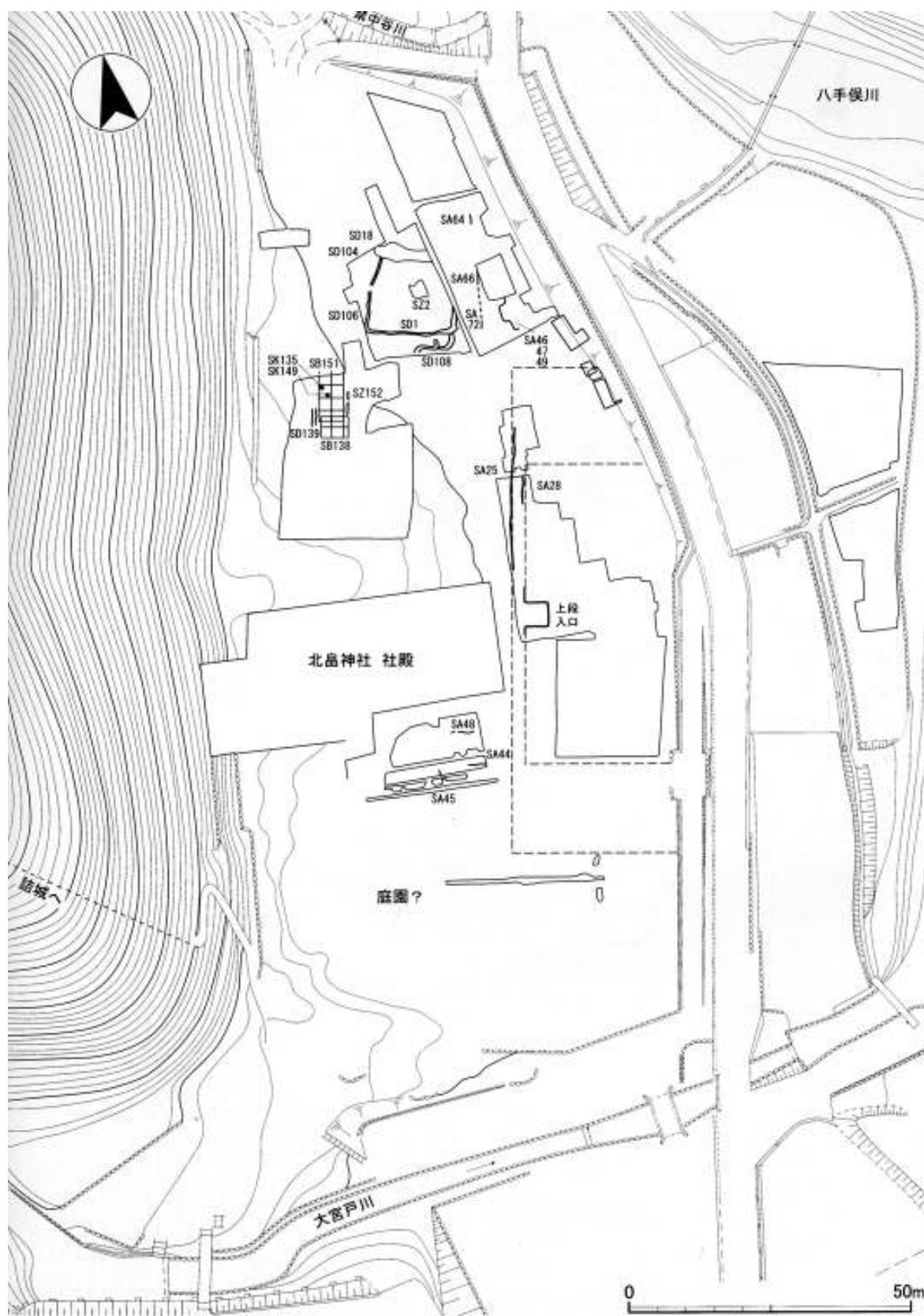
第2-6図 北畠氏館跡前期遺構図 (1:1,000)
