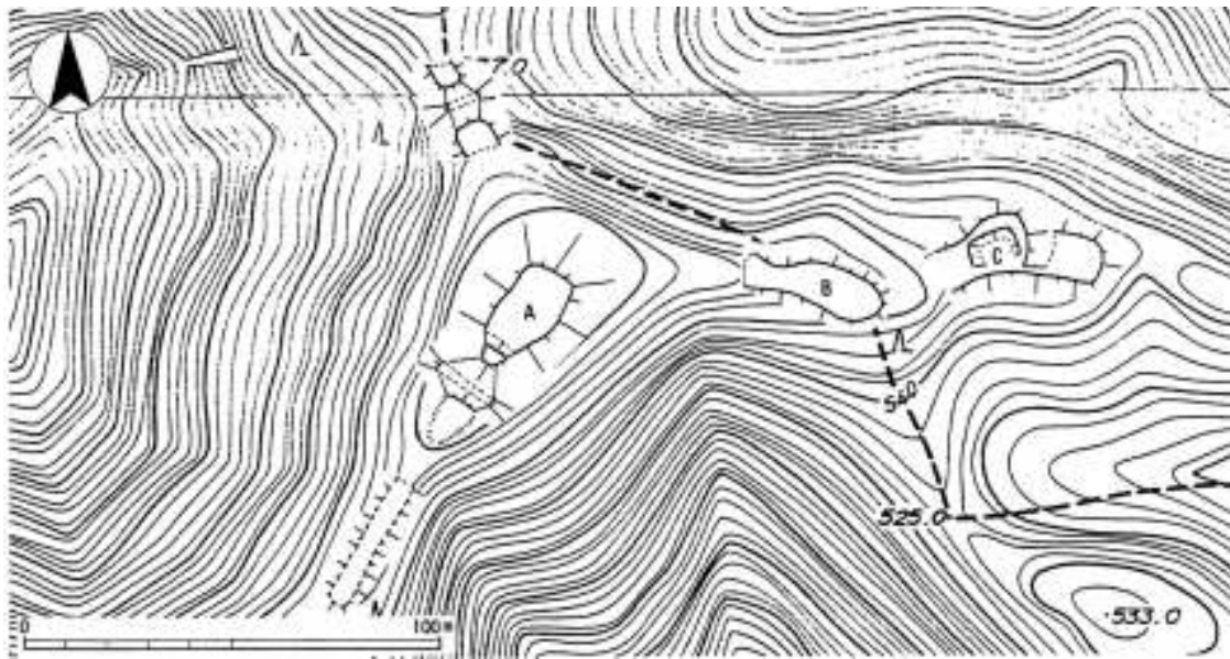
第2-10図 霧山城跡略測図（上：北曲輪郡、下：南曲輪郡、1：200 竹田憲治「中世北畠氏関連の城郭群－雲出川上流域を中心に－」『ミエヒストリー』11、2000年より転載）
