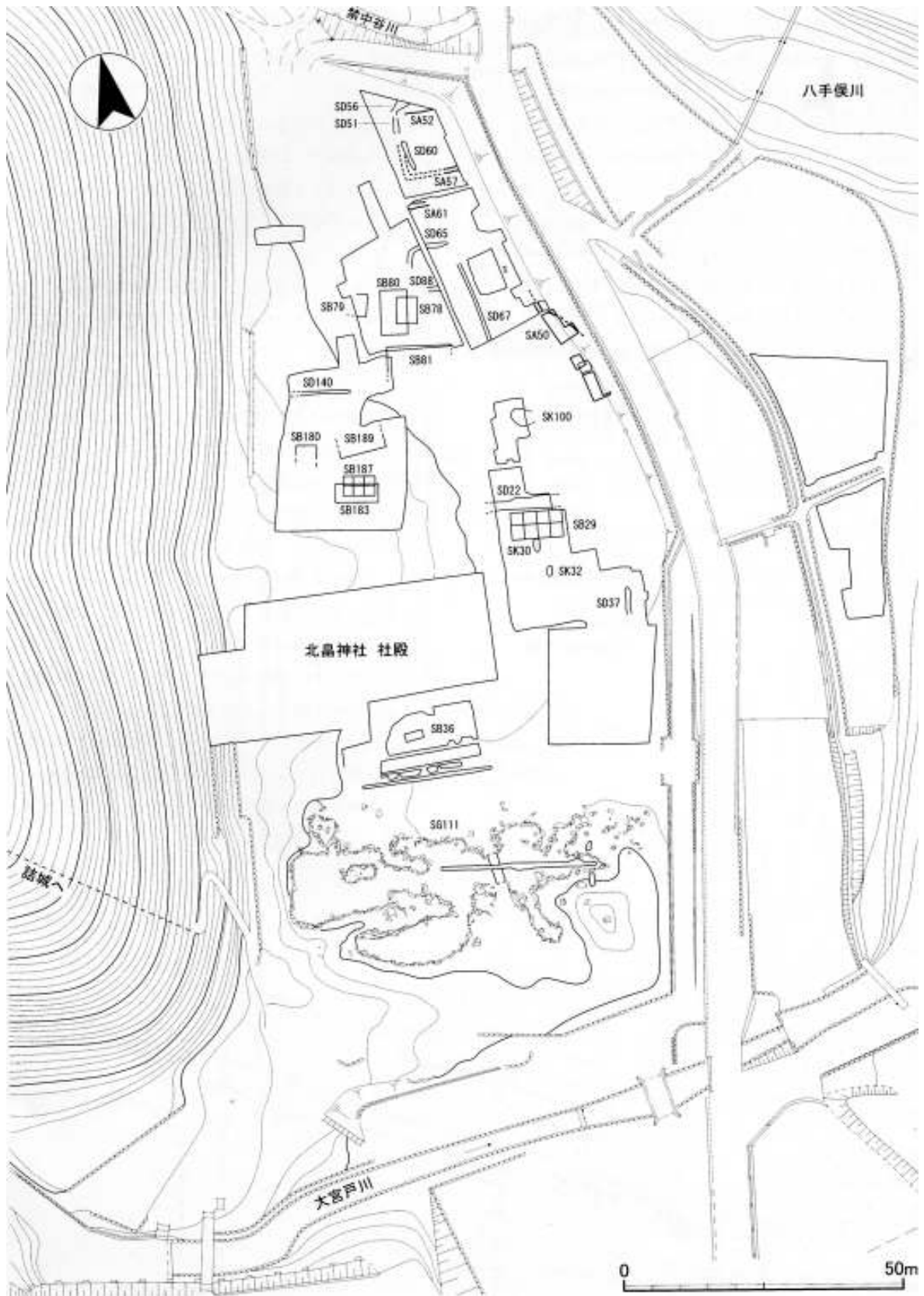
第2-7図 北畠氏館跡後期遺構図 (1:1,000)
