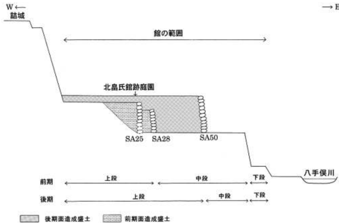
第2-8図 北畠氏館跡基礎構造概念図（縮尺不同）
