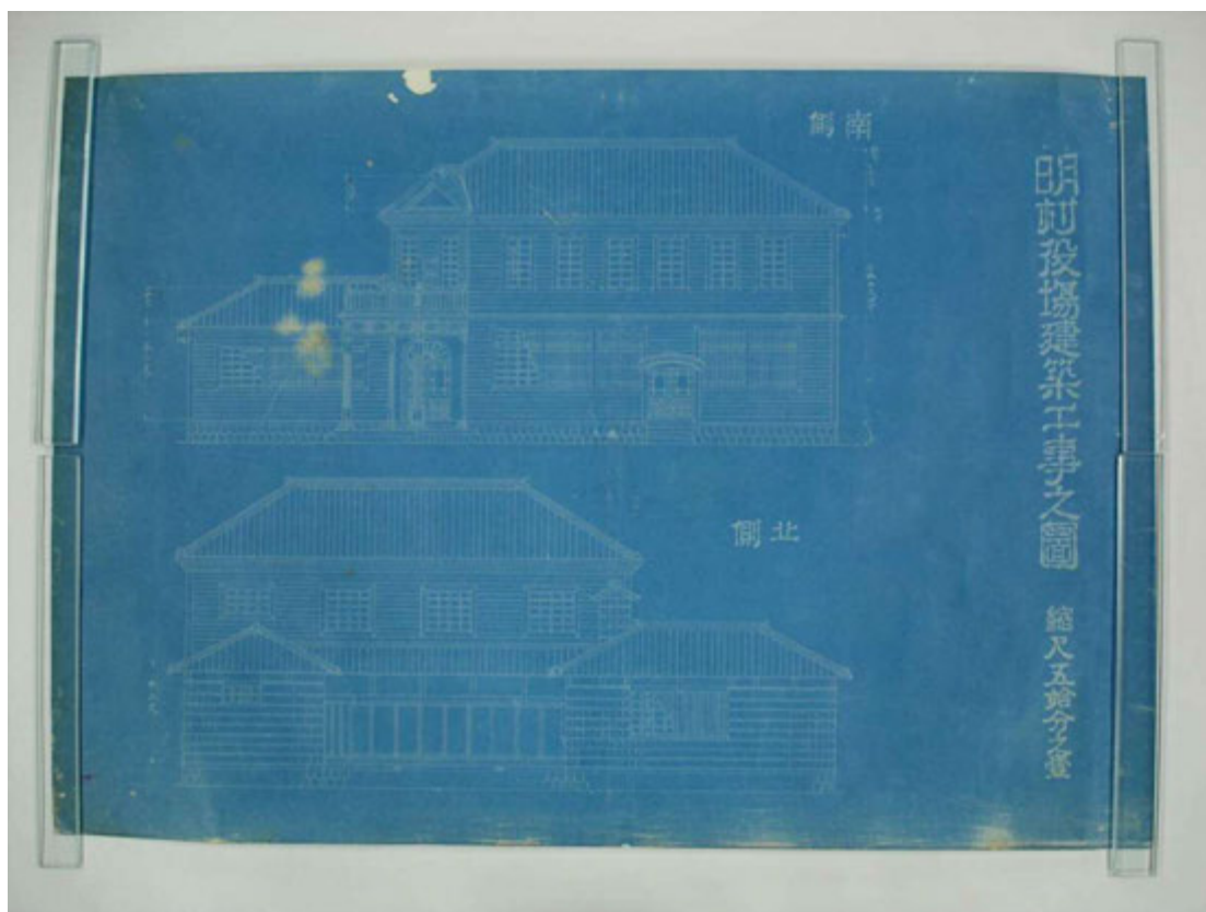
明村役場設計図①（南側立面・北側立面 1/50）
