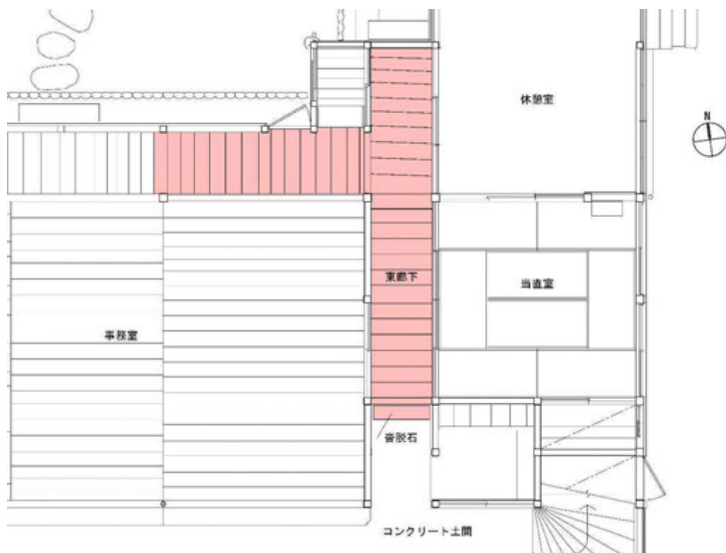
図 4-3 事務室東廊下の当初床板図
