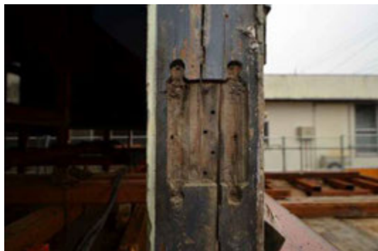
写真 4-5 自由蝶番の痕跡
