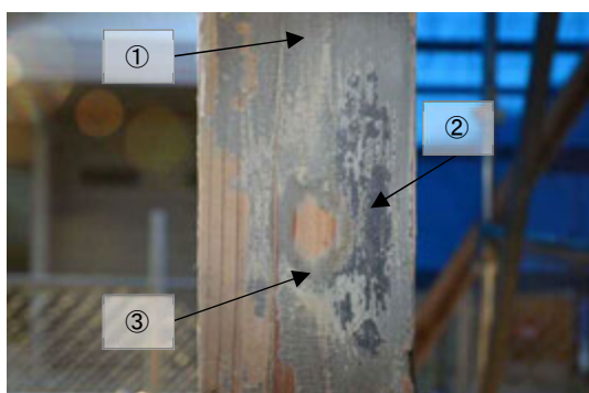
写真 3-4 来賓室棟の出入口脇柱の塗膜層
