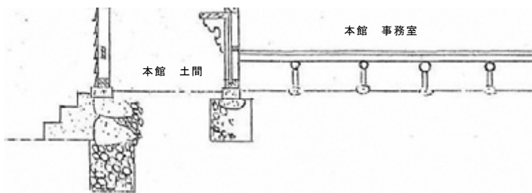
図 2-2 石積断面図 (A-A' 断面図)
