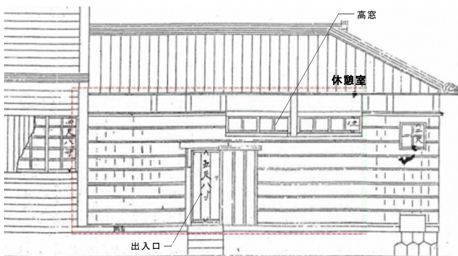
資料 4-2 東立面図（当初設計図より）
