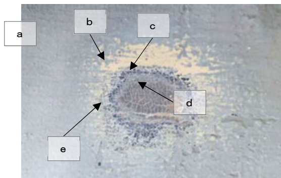
写真 3-2 軒蛇腹の塗膜層
