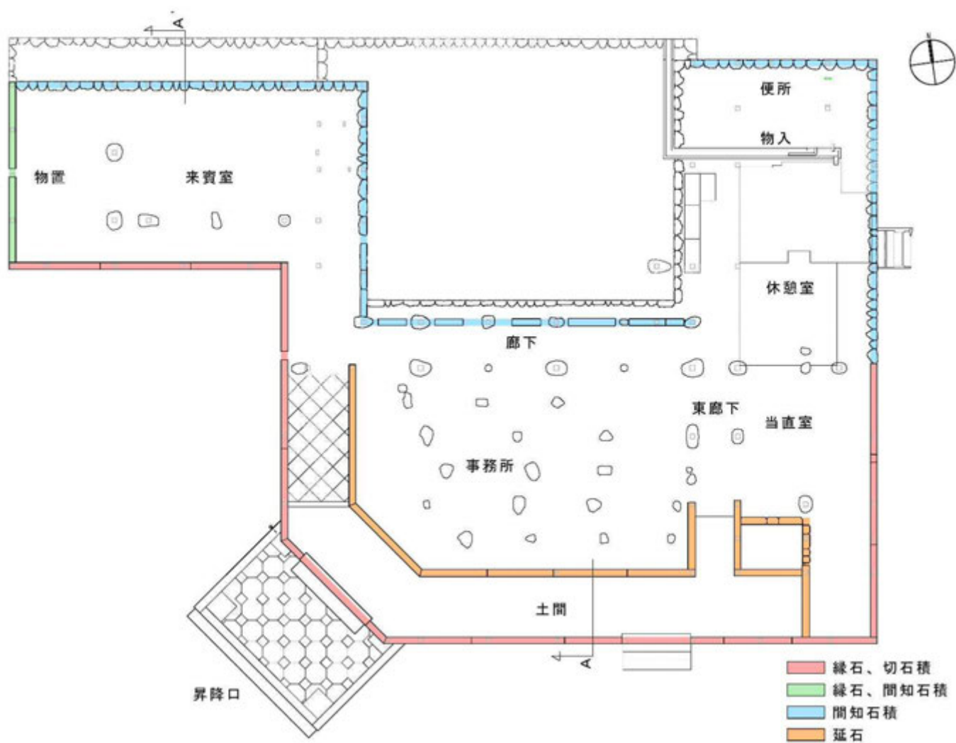
図 2-1 基礎伏図
