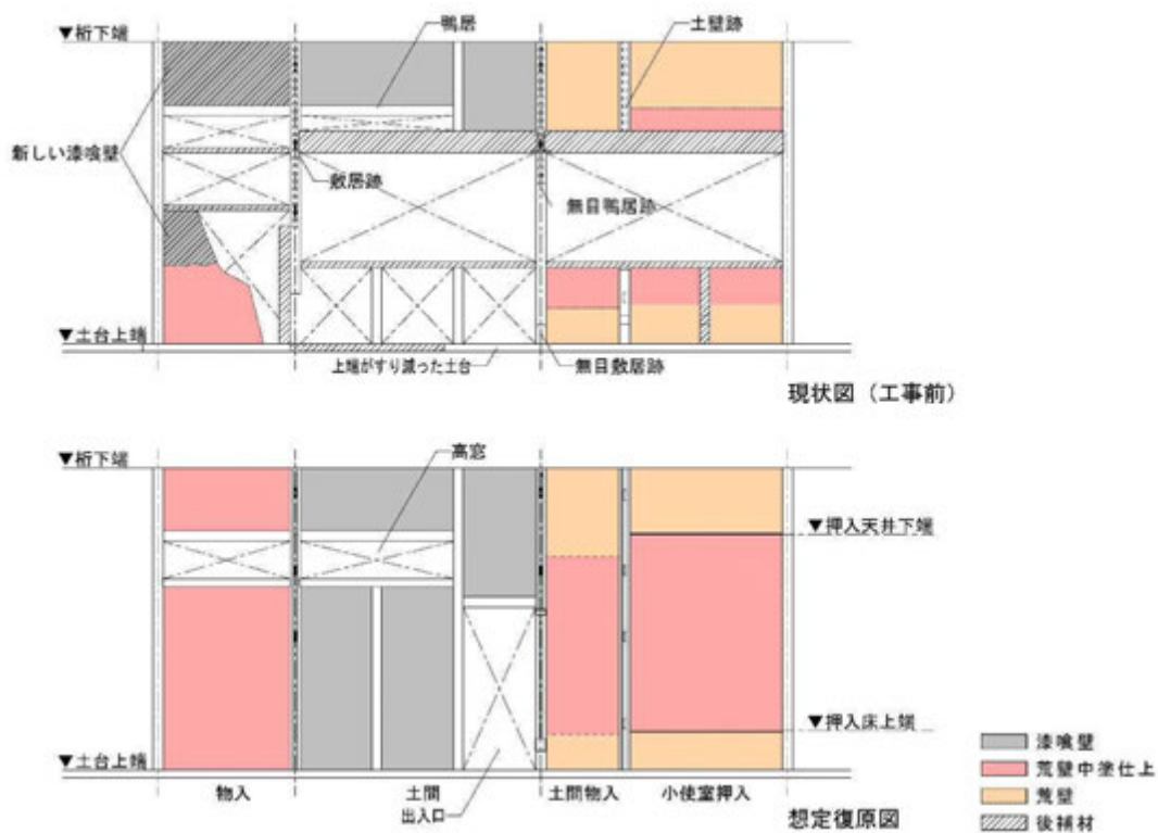
図 4-7 休憩室東面展開図
