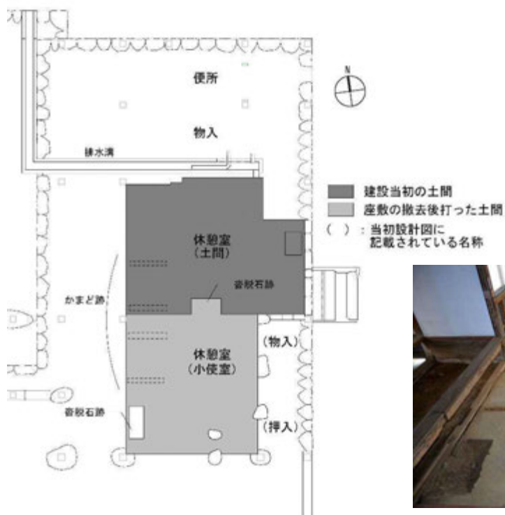
図 4-6 休憩室土間状況図
