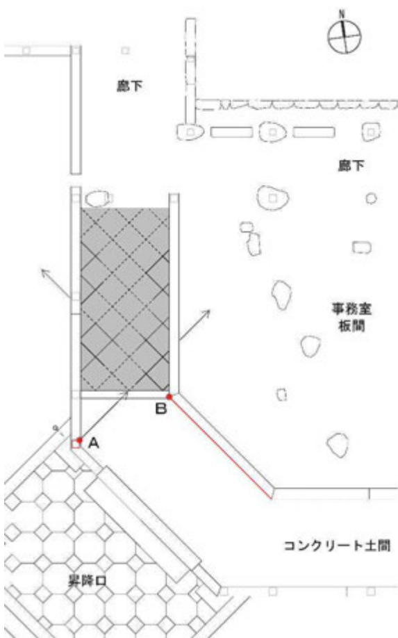
図 4-2 事務室西側 四半目地土間状況図
