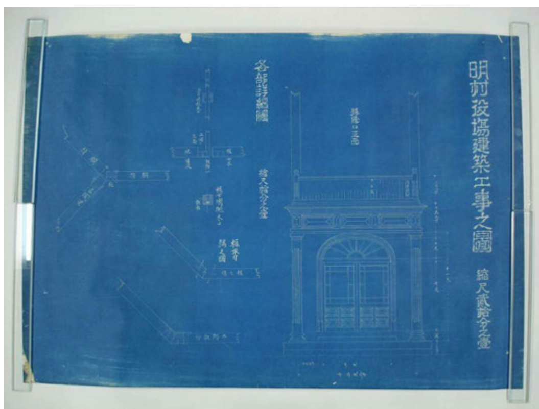
明村役場設計図⑥（各館詳細図 1/20）
