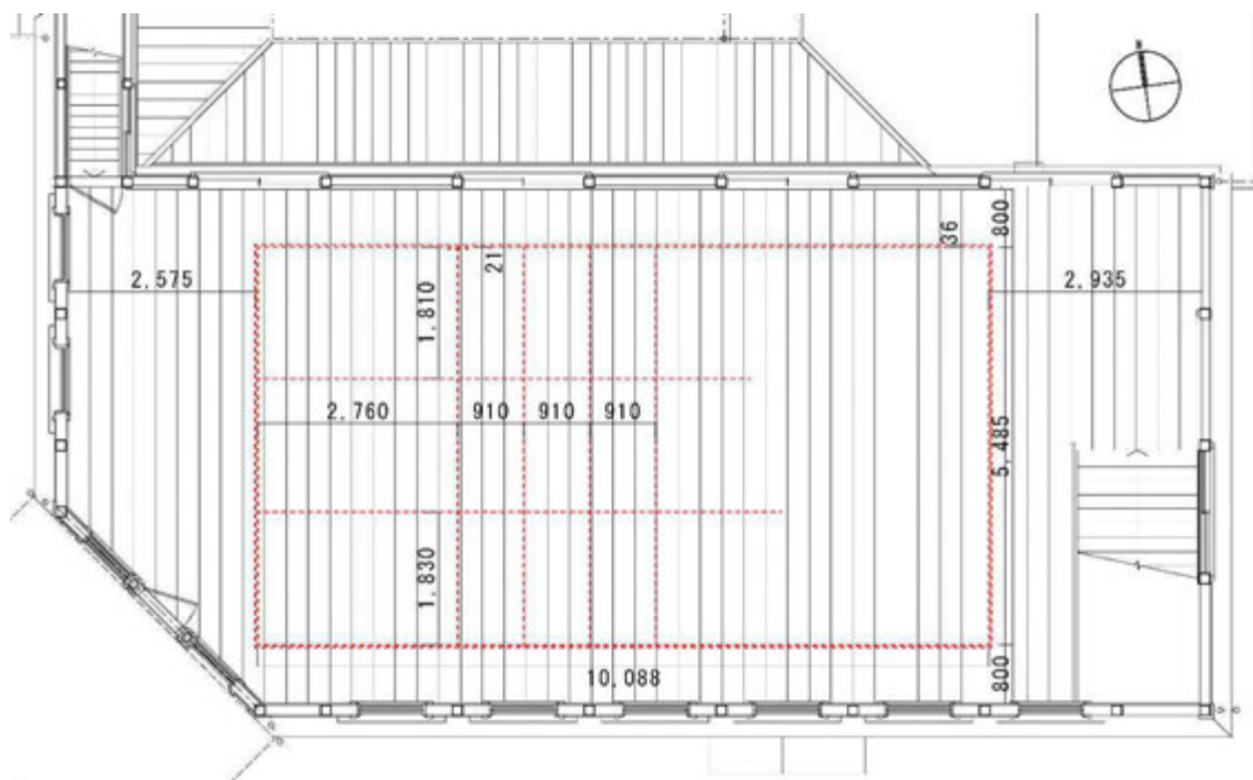
図 4-5 議場 畳敷き痕跡図
