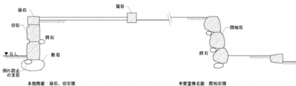
図 2-2 石積断面図 (A-A' 断面図)
