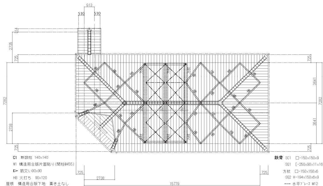
屋根伏図
