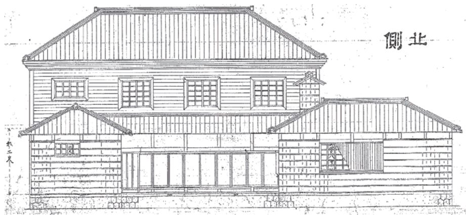
（大正５年建設当初図面）
