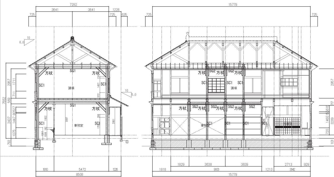
梁間断面図
