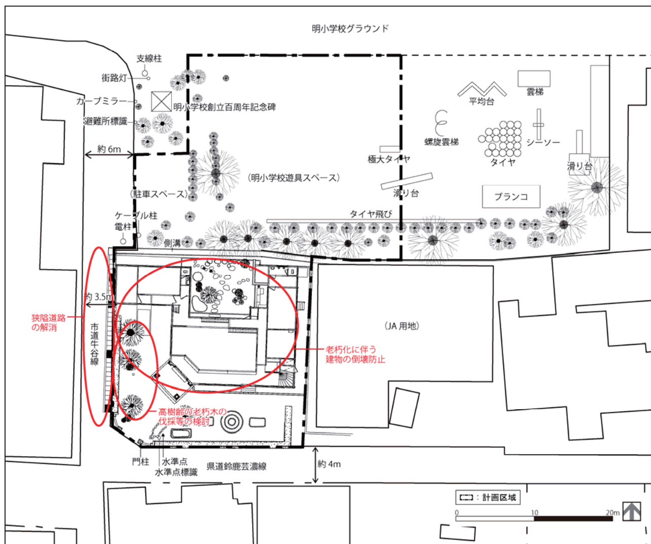
圖一 課題圖
