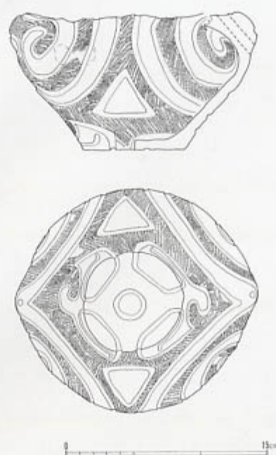
遺物実測図 (1:4)
