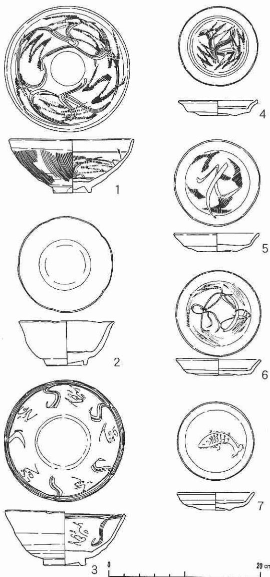
青磁碗・小皿実測図 (1:5)
