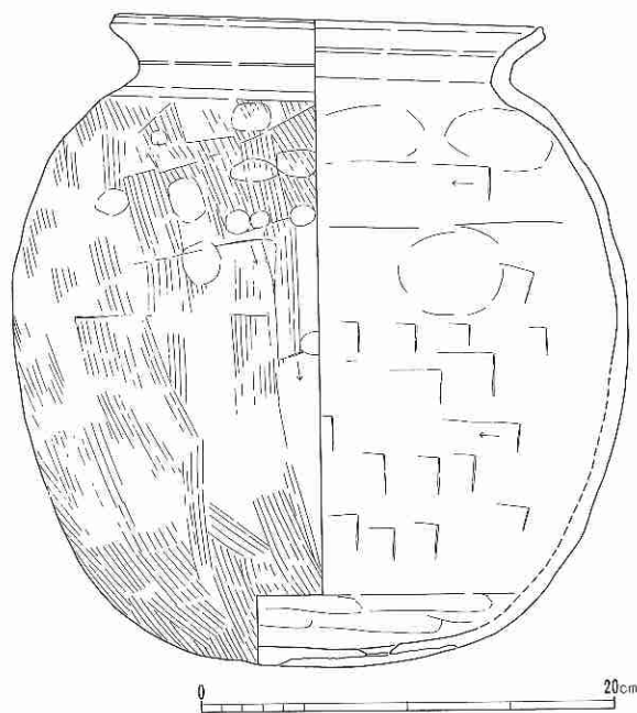
遺物実測図(1:4)
