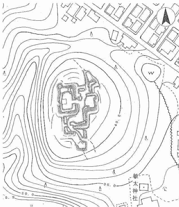
宮山城跡実測図
